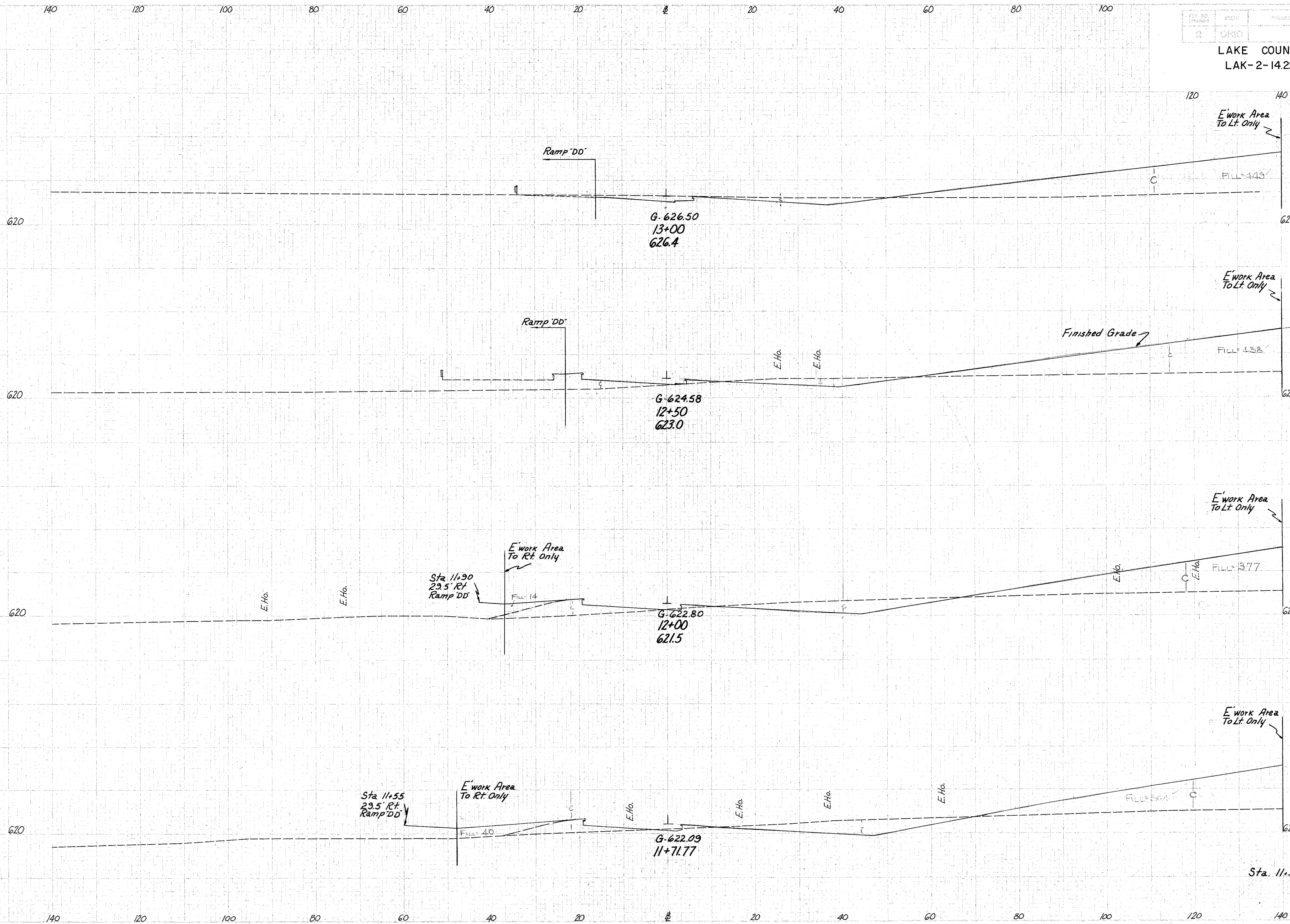
Ramp C-C Sta. 11+71.77 to Sta. 13+00
