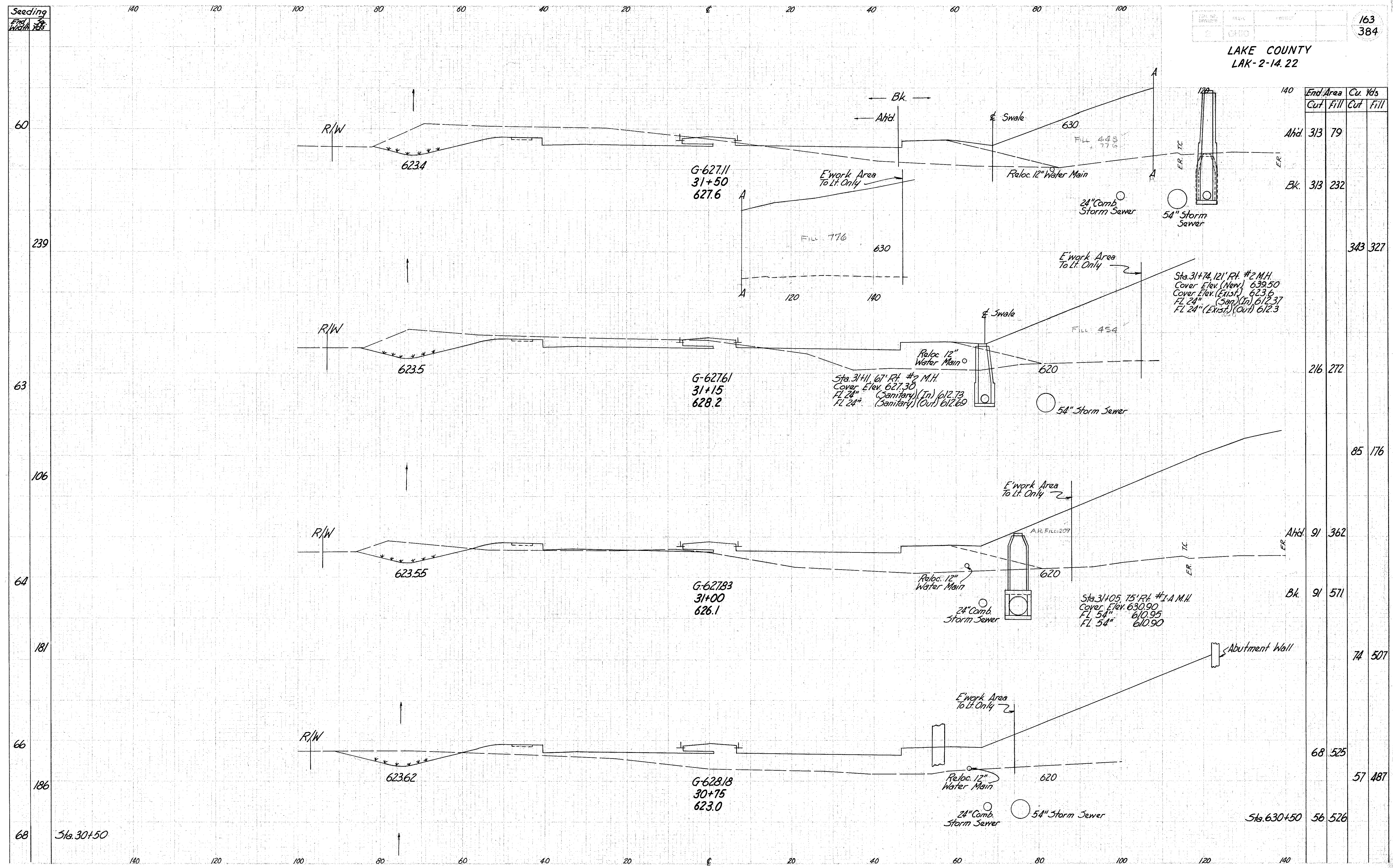
Reloc. Richmond St. Sta. 30+75 to Sta. 31+50
