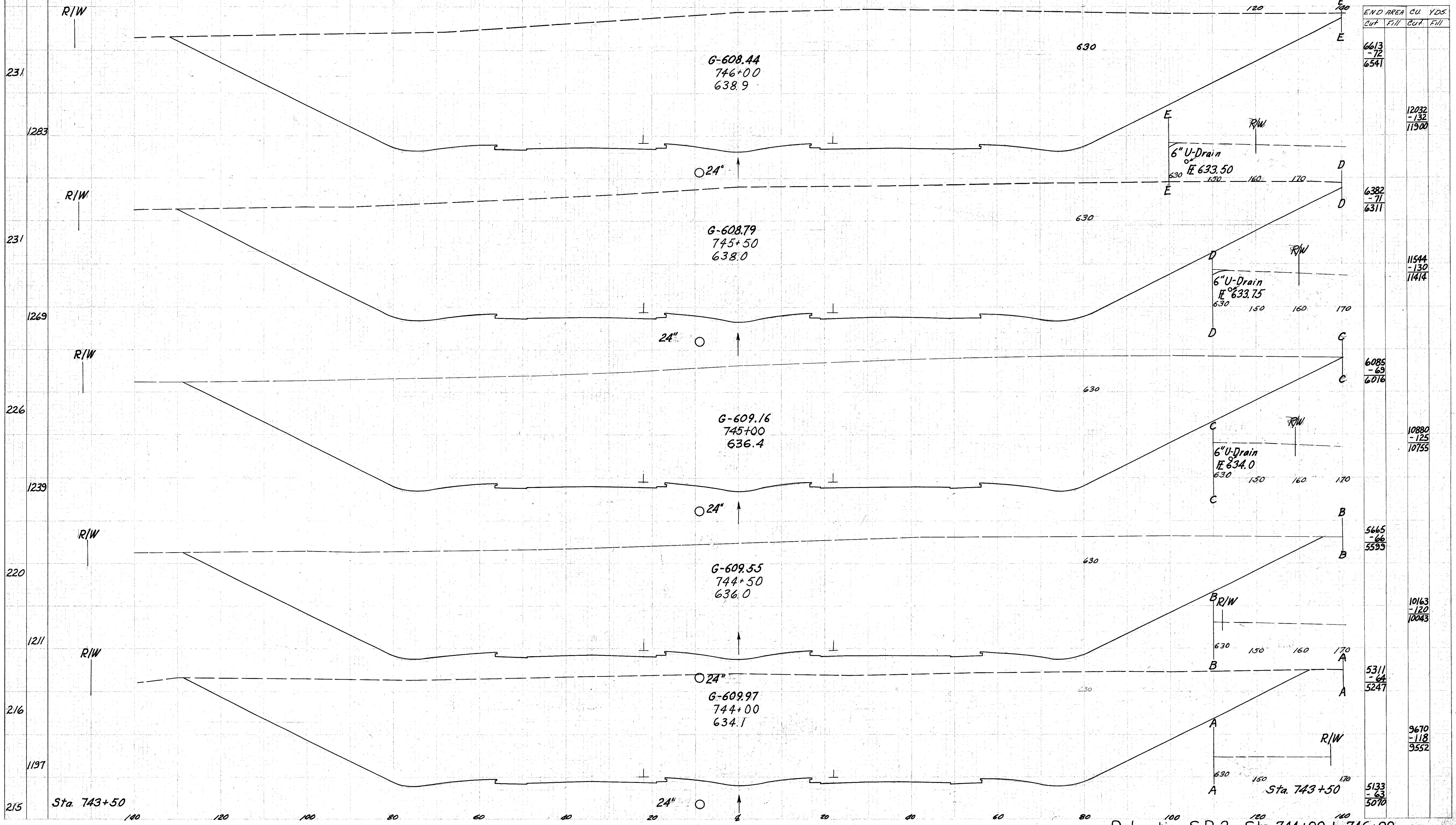
Relocation S.R.2 Sta. 744+00 to 746+00
