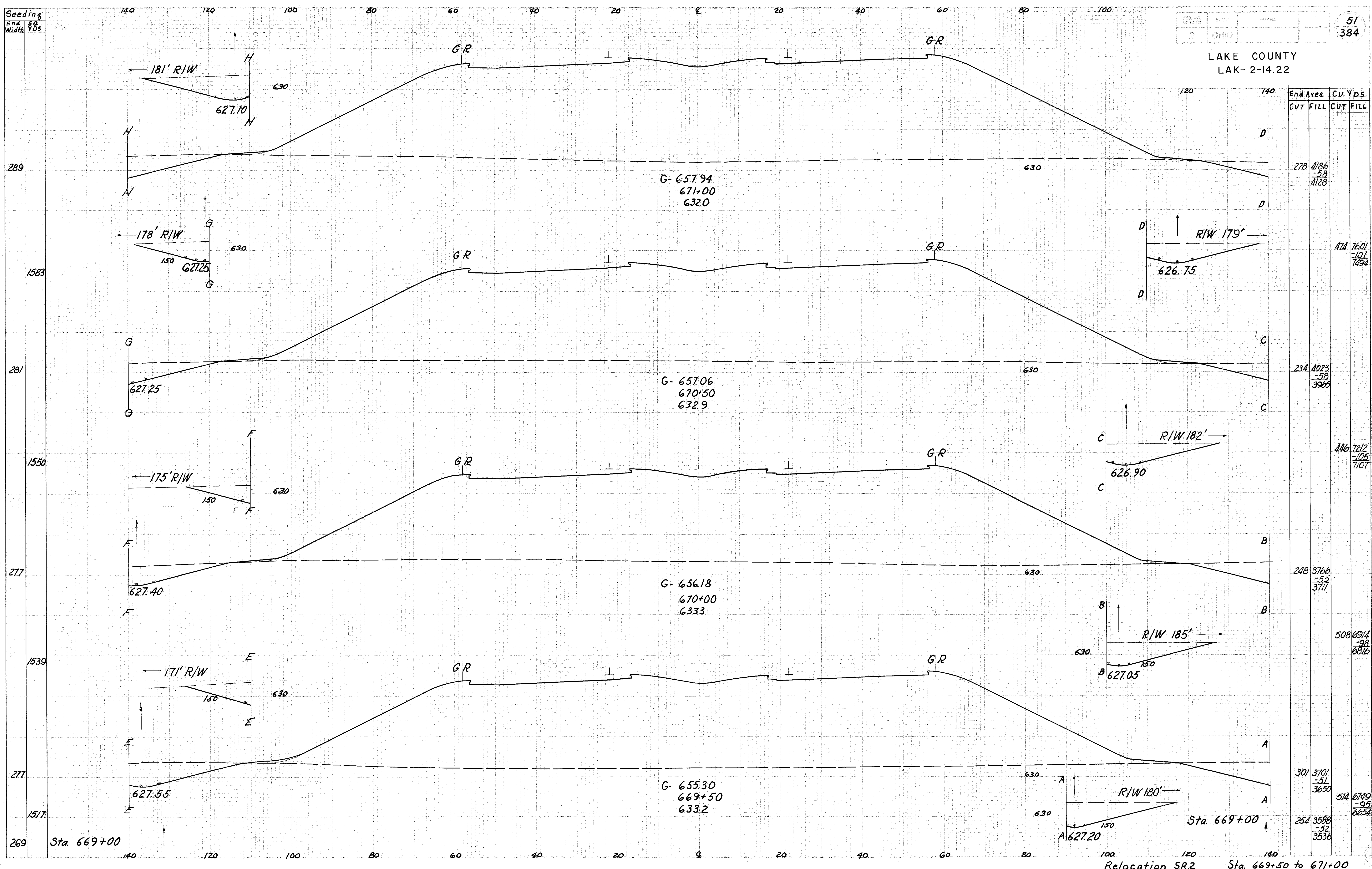
Relocation SR2 Sta. 669+50 to 671+00
