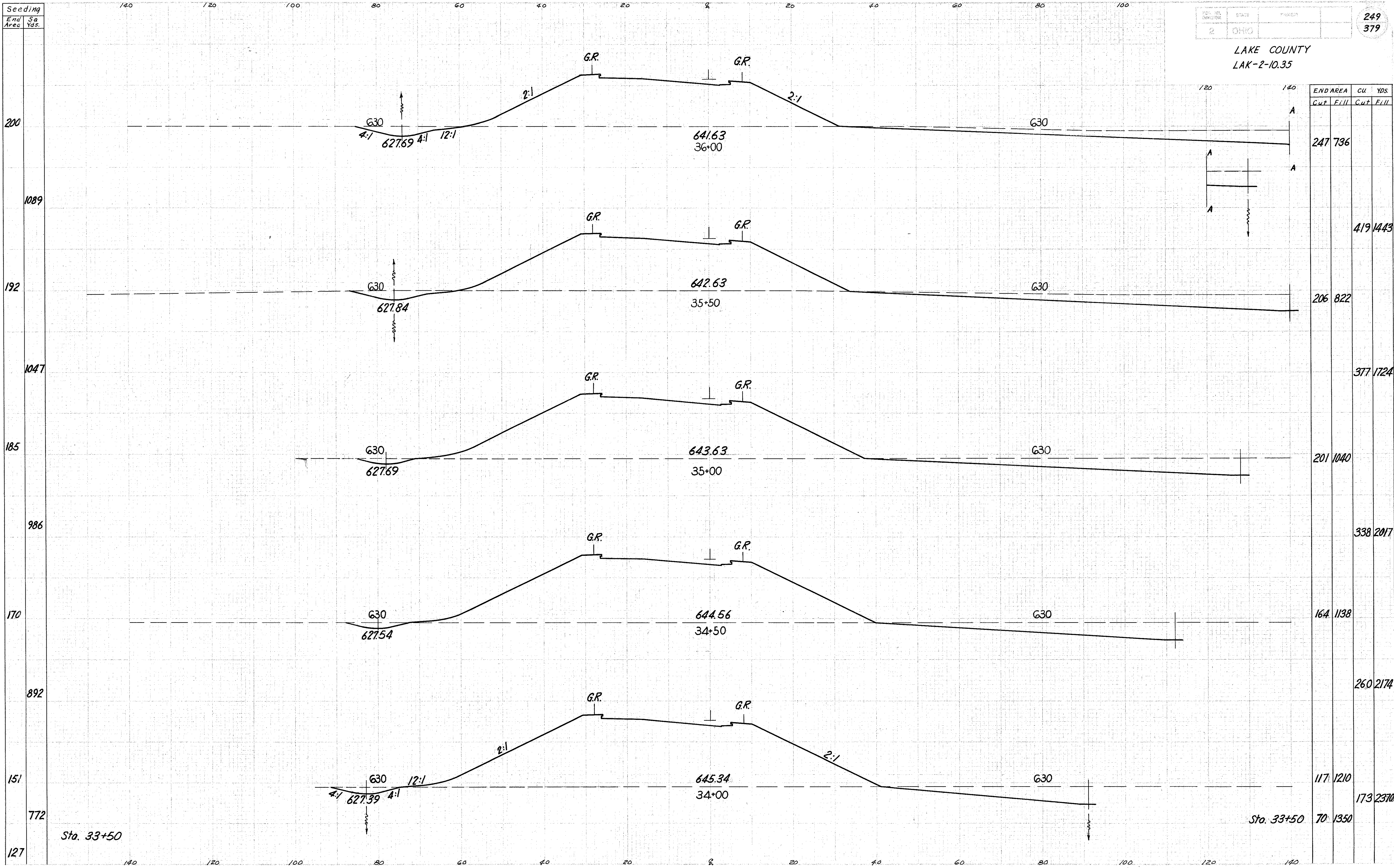
Ramp G Sta. 34+00 to 36+00
