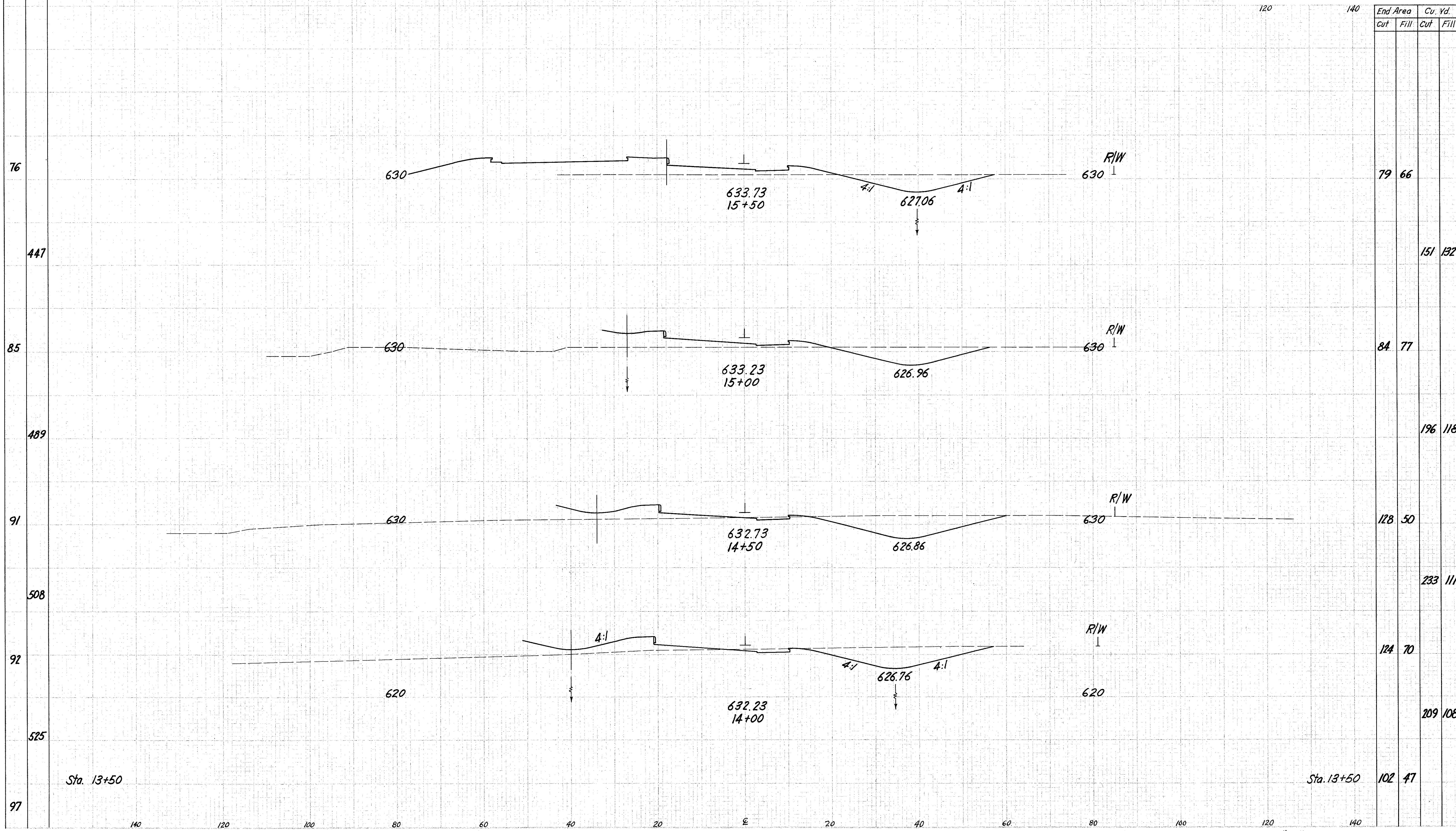
Ramp "F" Sta. 14+00 to 15+50
