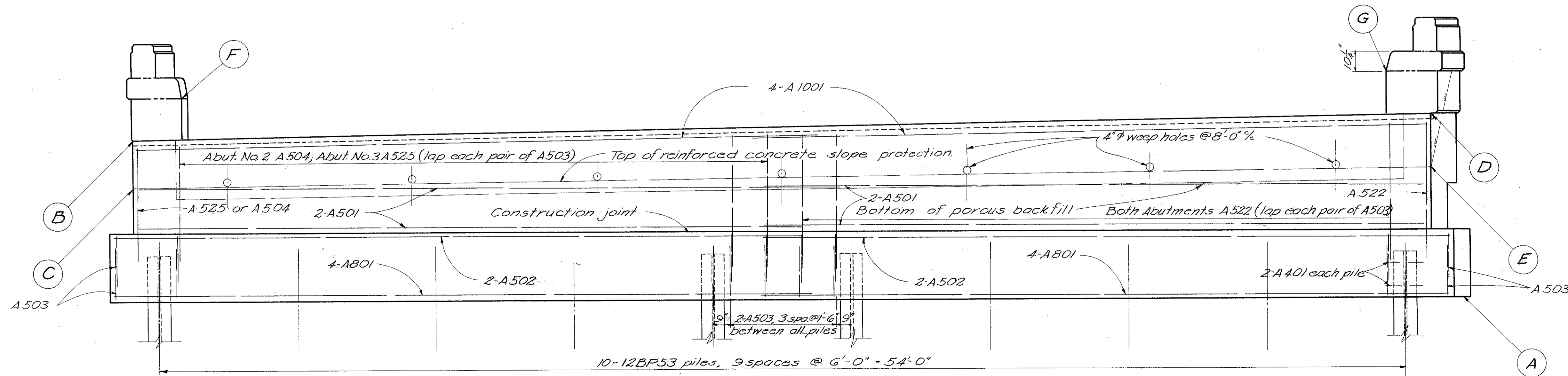
ELEVATION
