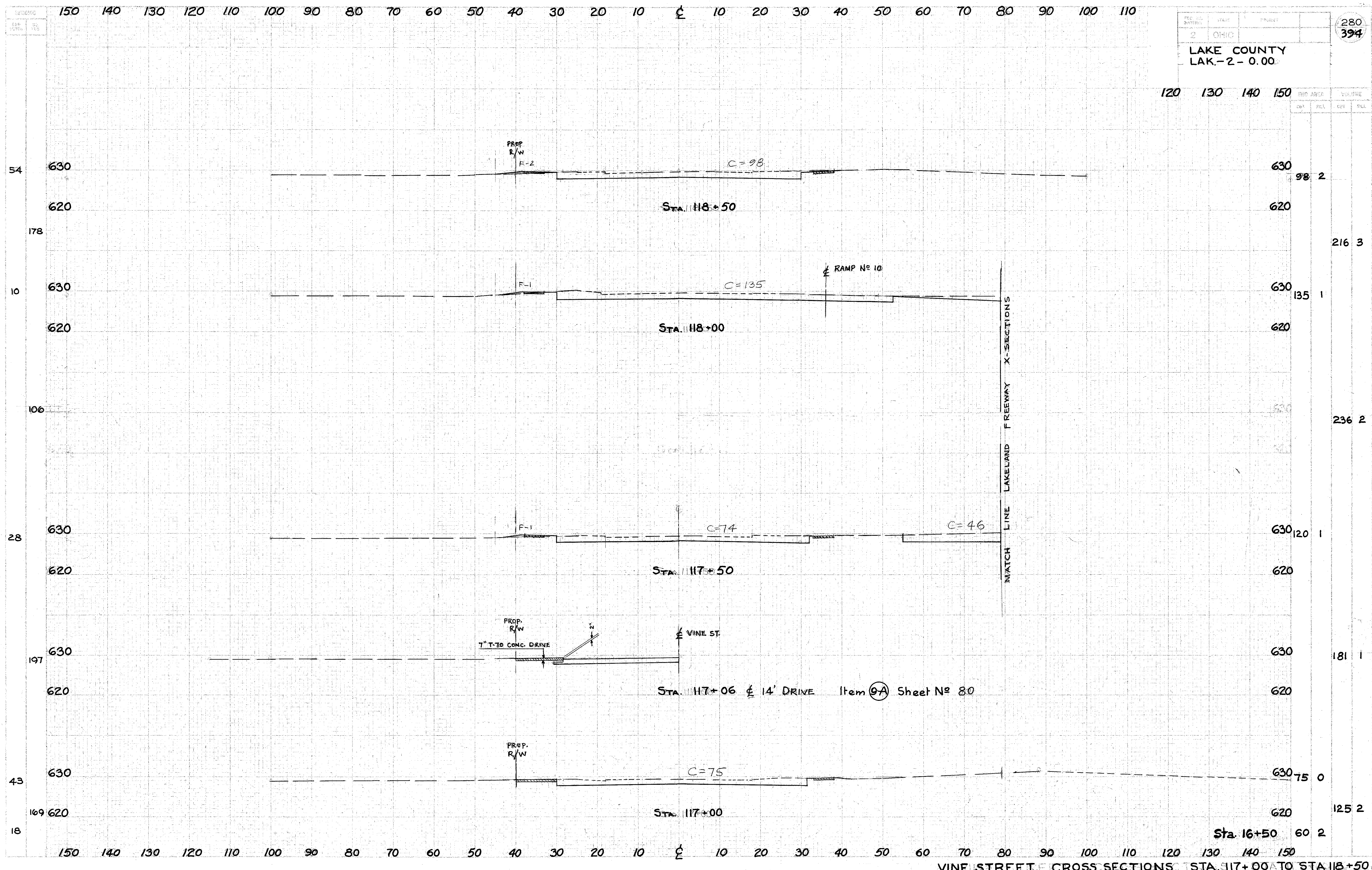
VINE STREET CROSS SECTIONS STA. 117+00 TO STA. 118+50
