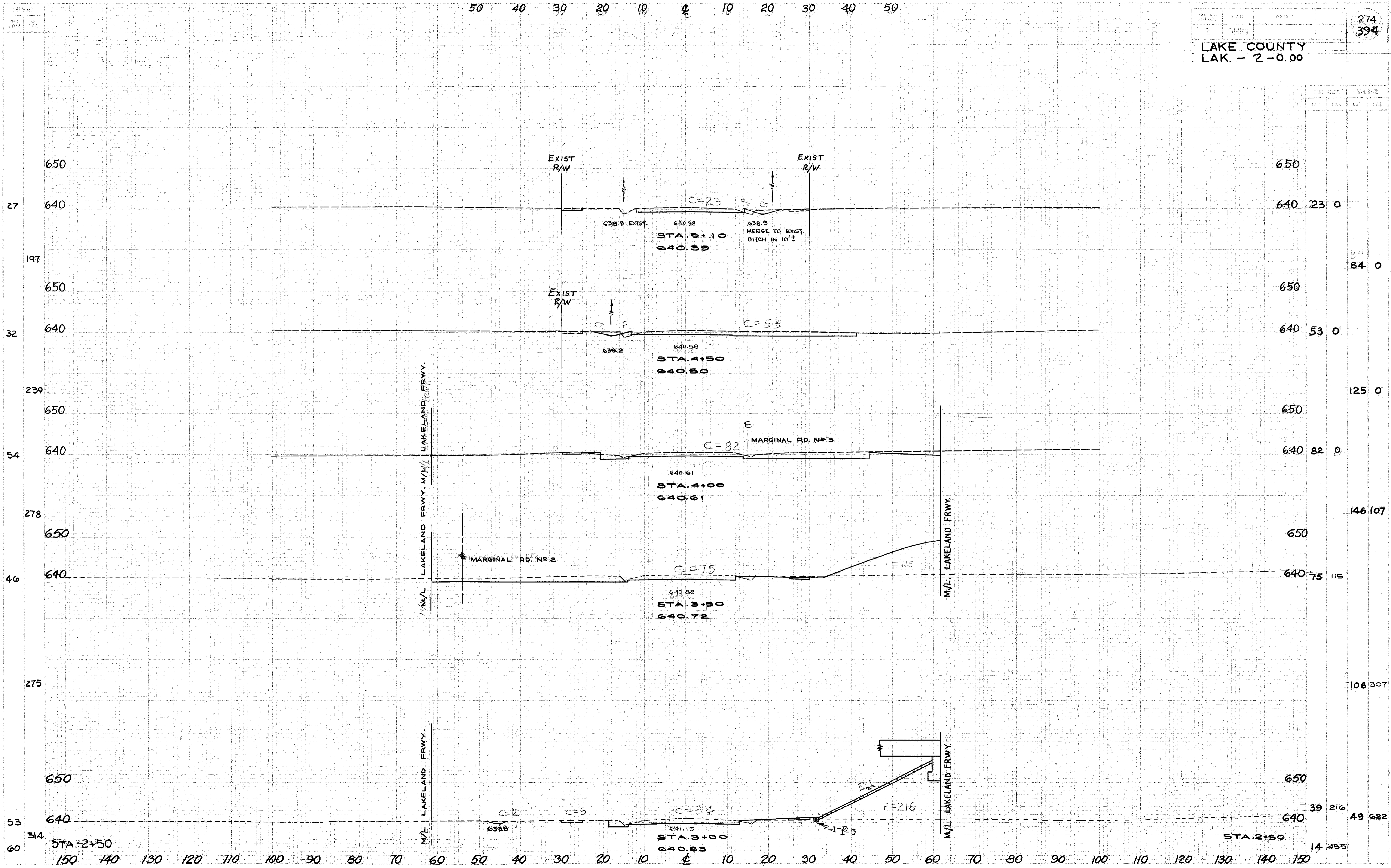
CAMPBELL RD. (E 337) CROSS SECTIONS STA. (3+00 TO STA. 5+10
