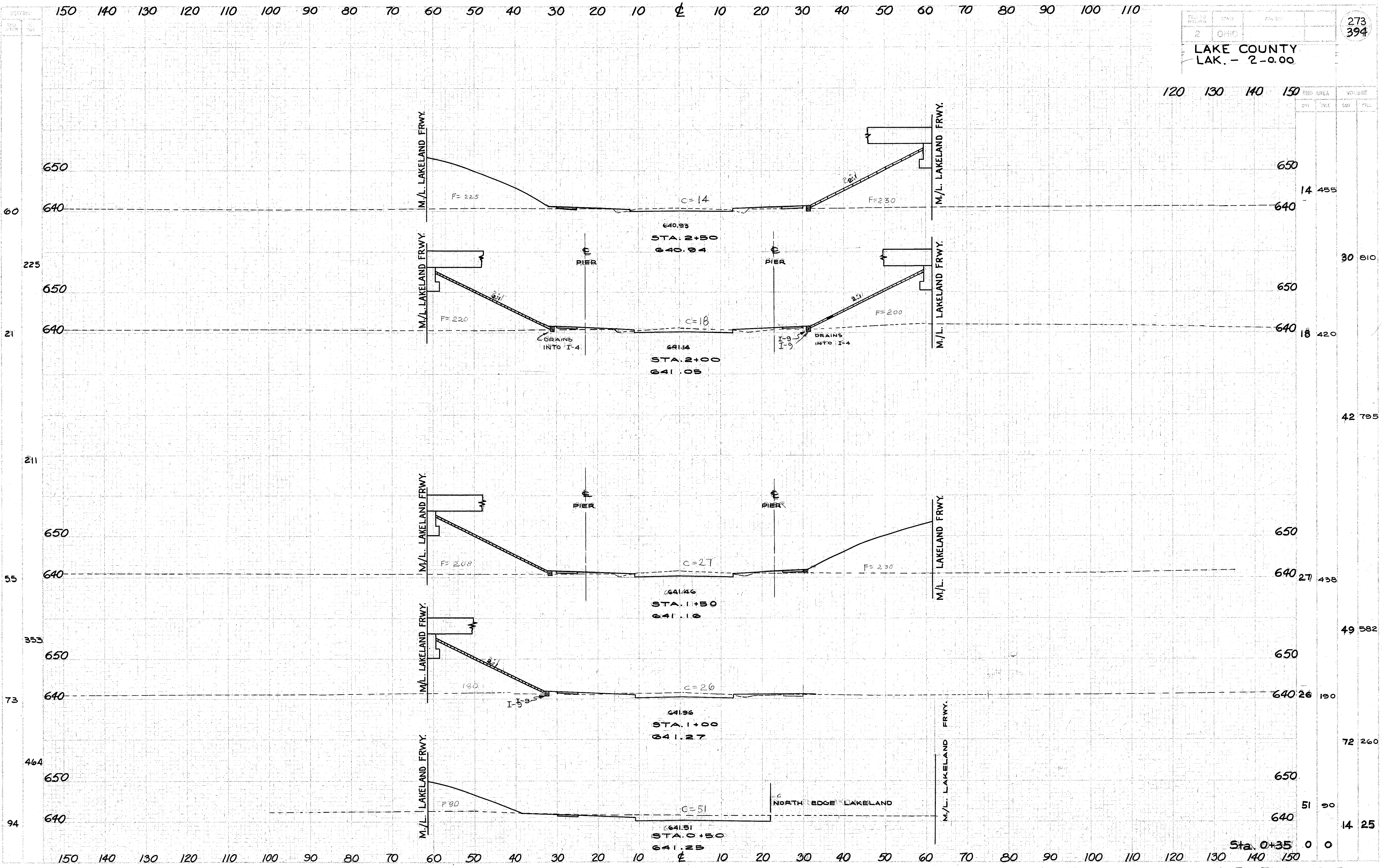
CAMPBELL RD. (E 337) CROSS SECTIONS STA. 0+50 TO STA. 2+50
