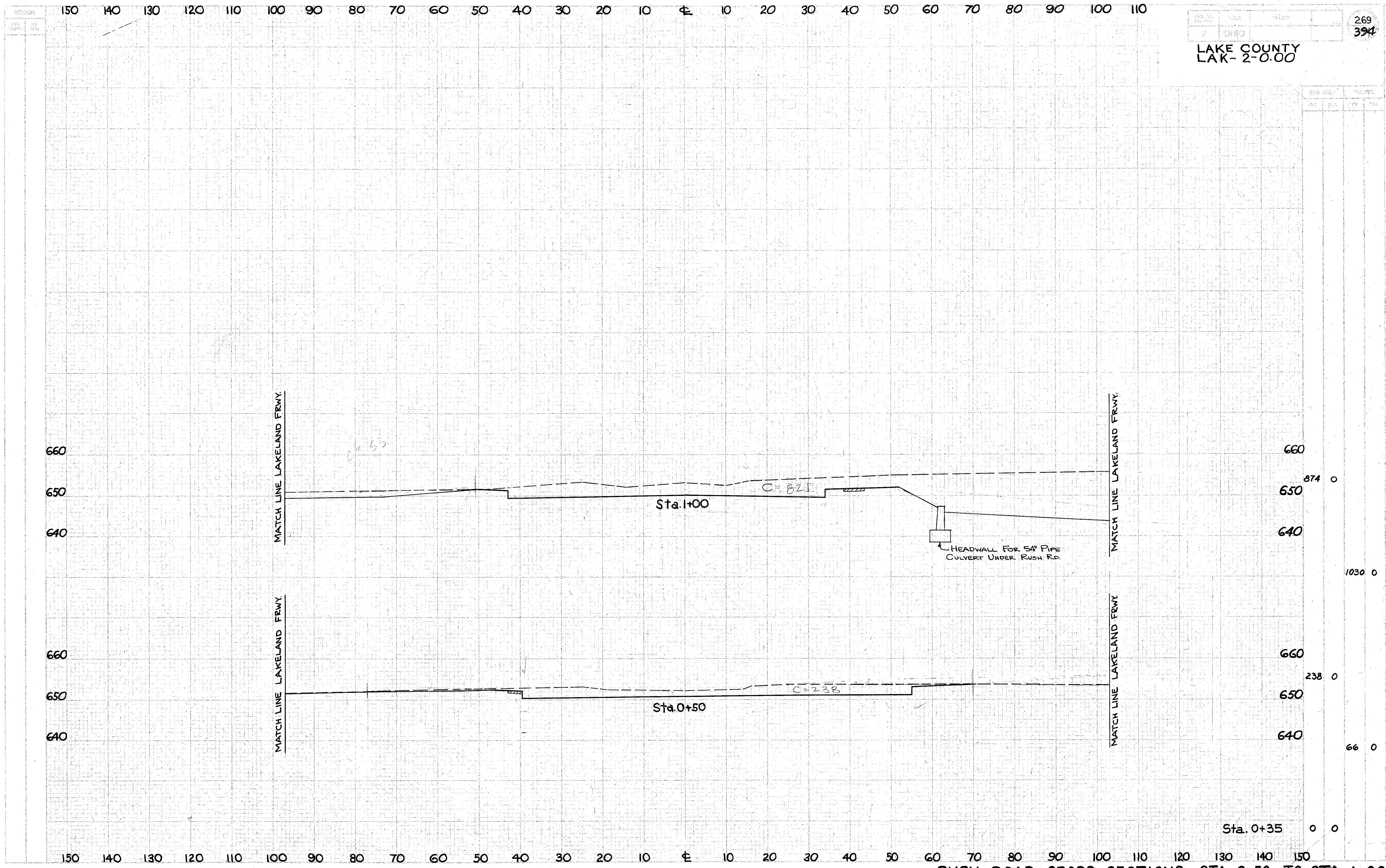
RUSH ROAD CROSS SECTIONS STA. 0+50 TO STA. 1+00
