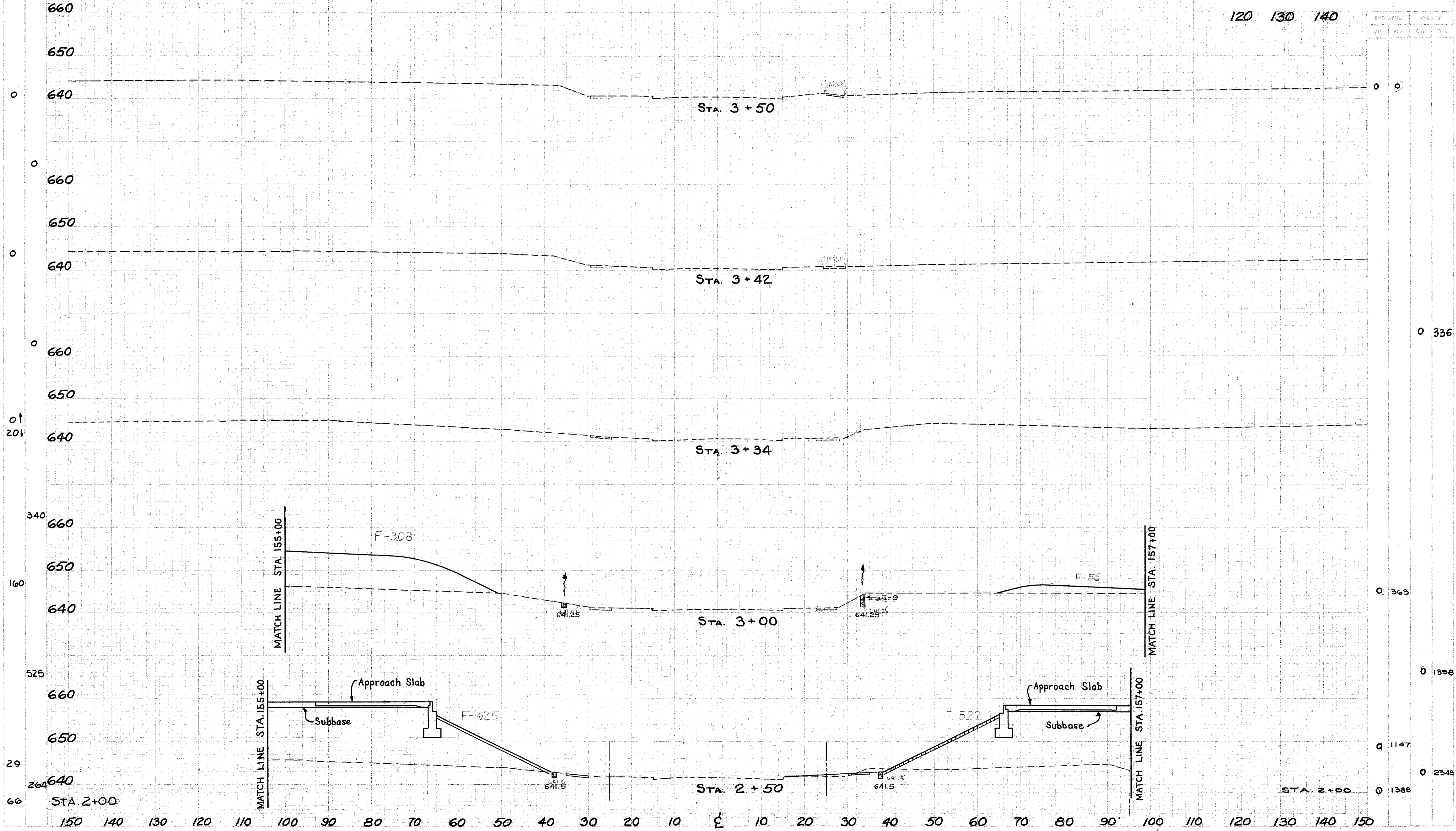
WORDEN RD. CROSS SECTIONS STA. 2+50 TO STA. 3+50
