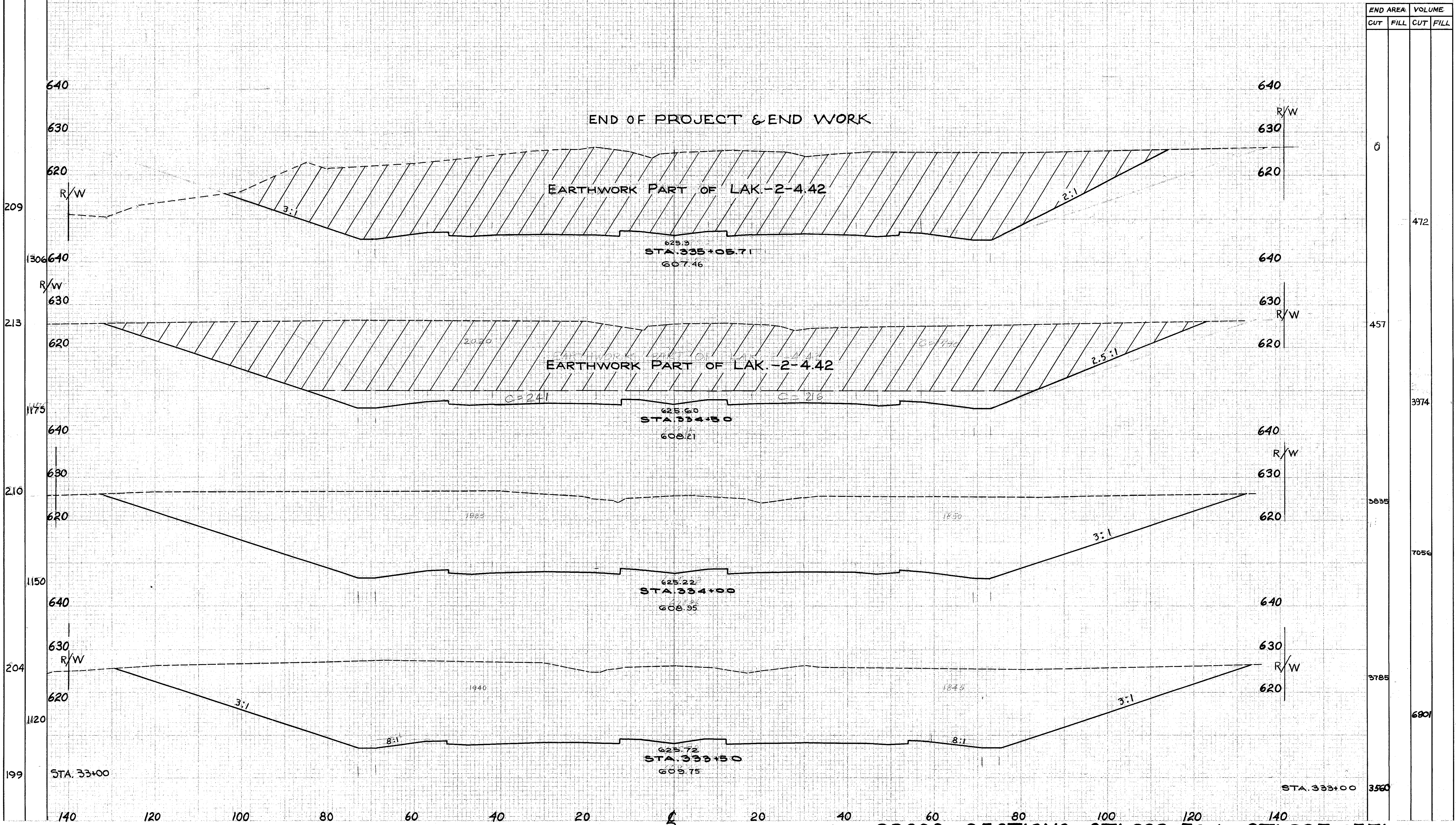
CROSS SECTIONS STA. 333+50 to STA. 335+05.71
