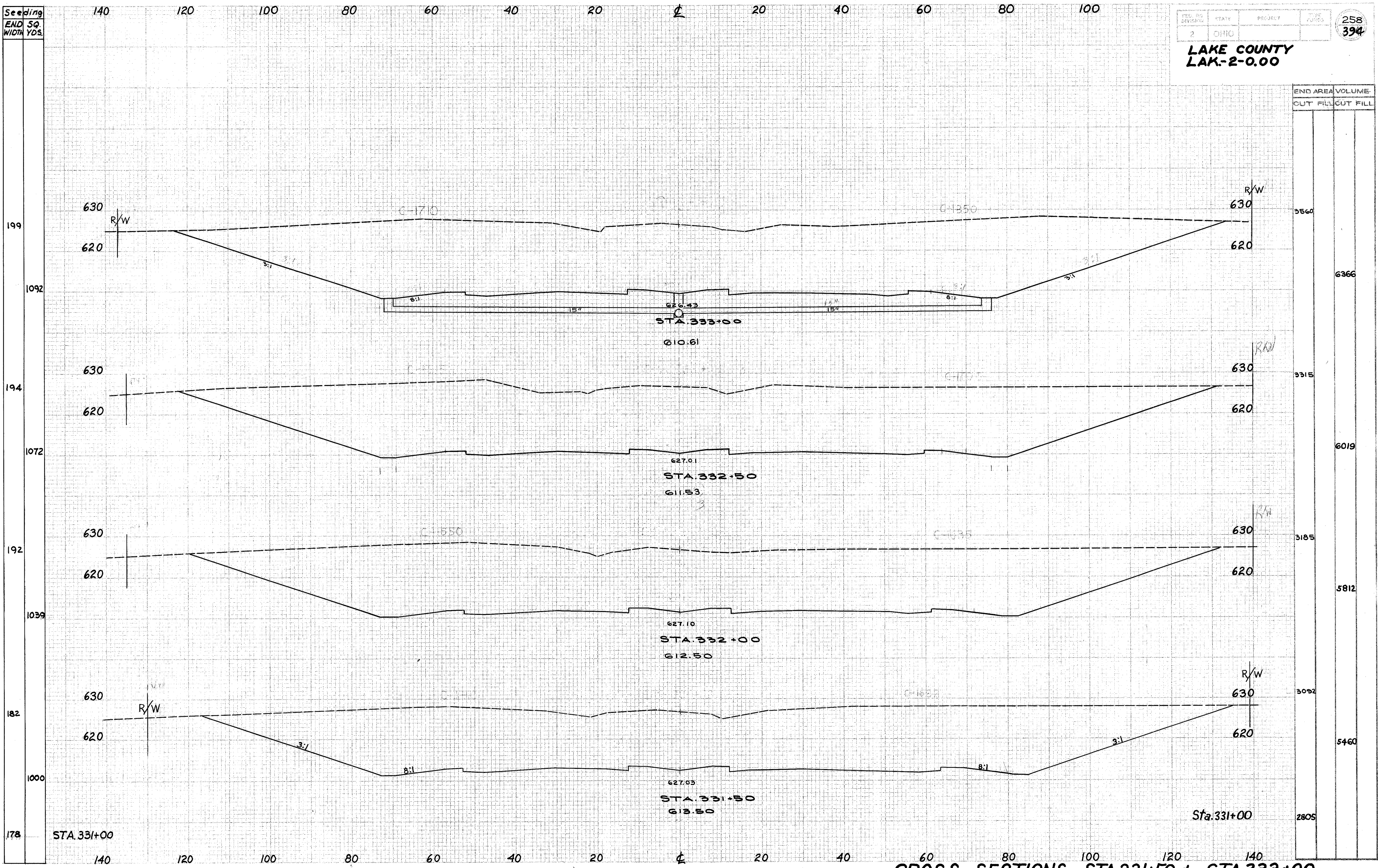
CROSS SECTIONS - STA. 331+50 to STA. 333+00
