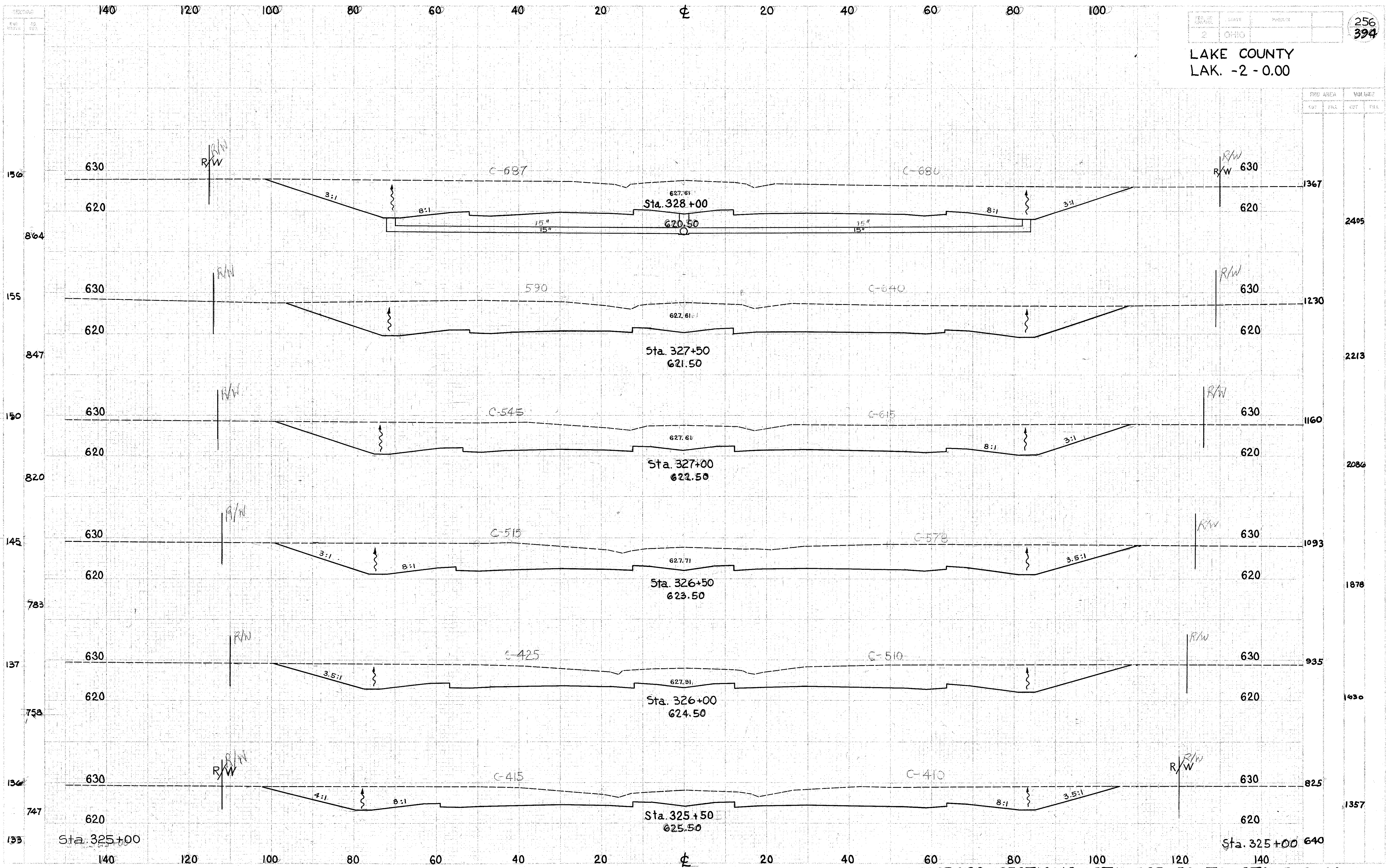
CROSS SECTIONS STA. 325+50 TO STA. 328+00
