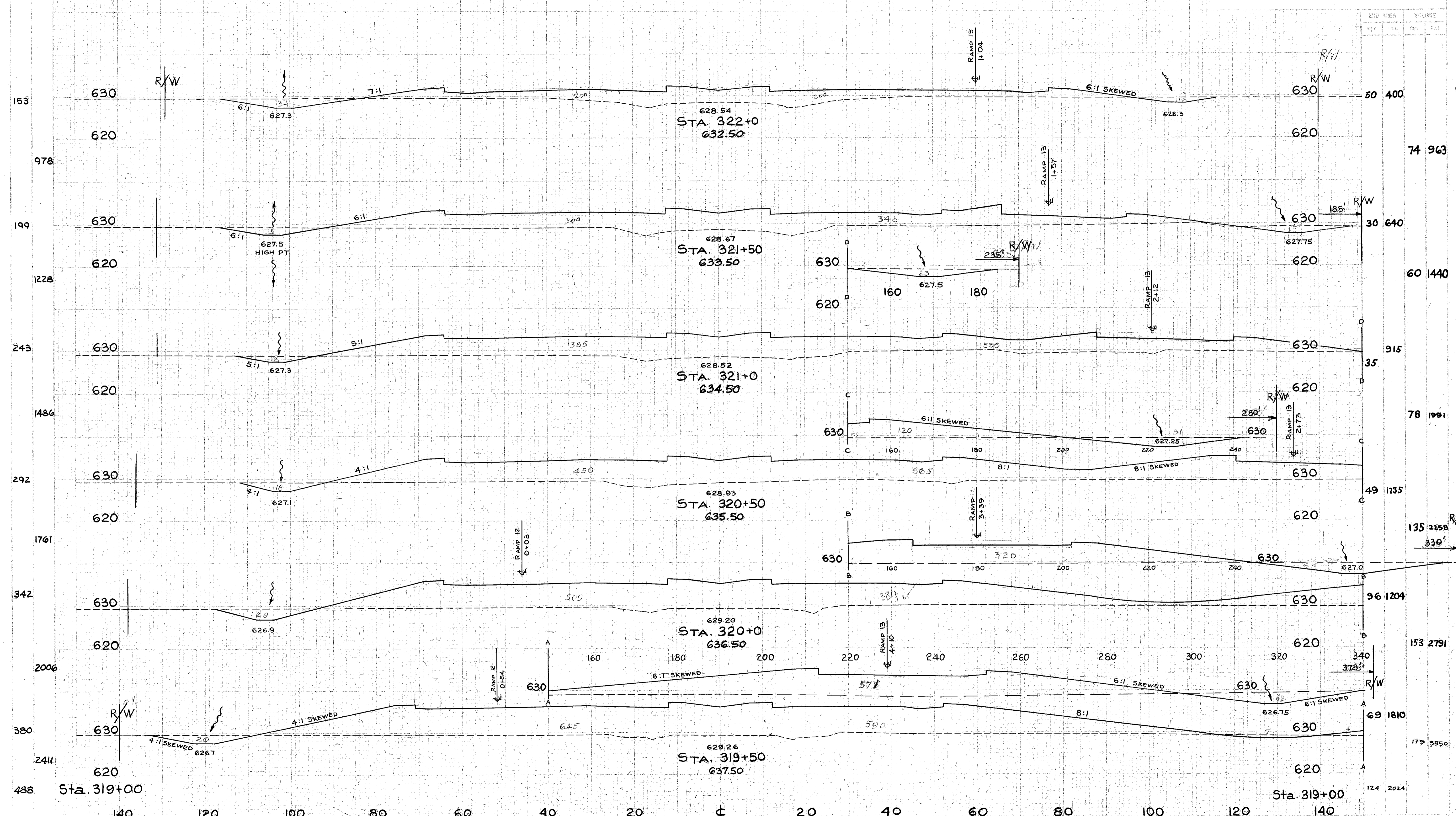
CROSS SECTIONS STA. 319+50 TO STA. 322+0
