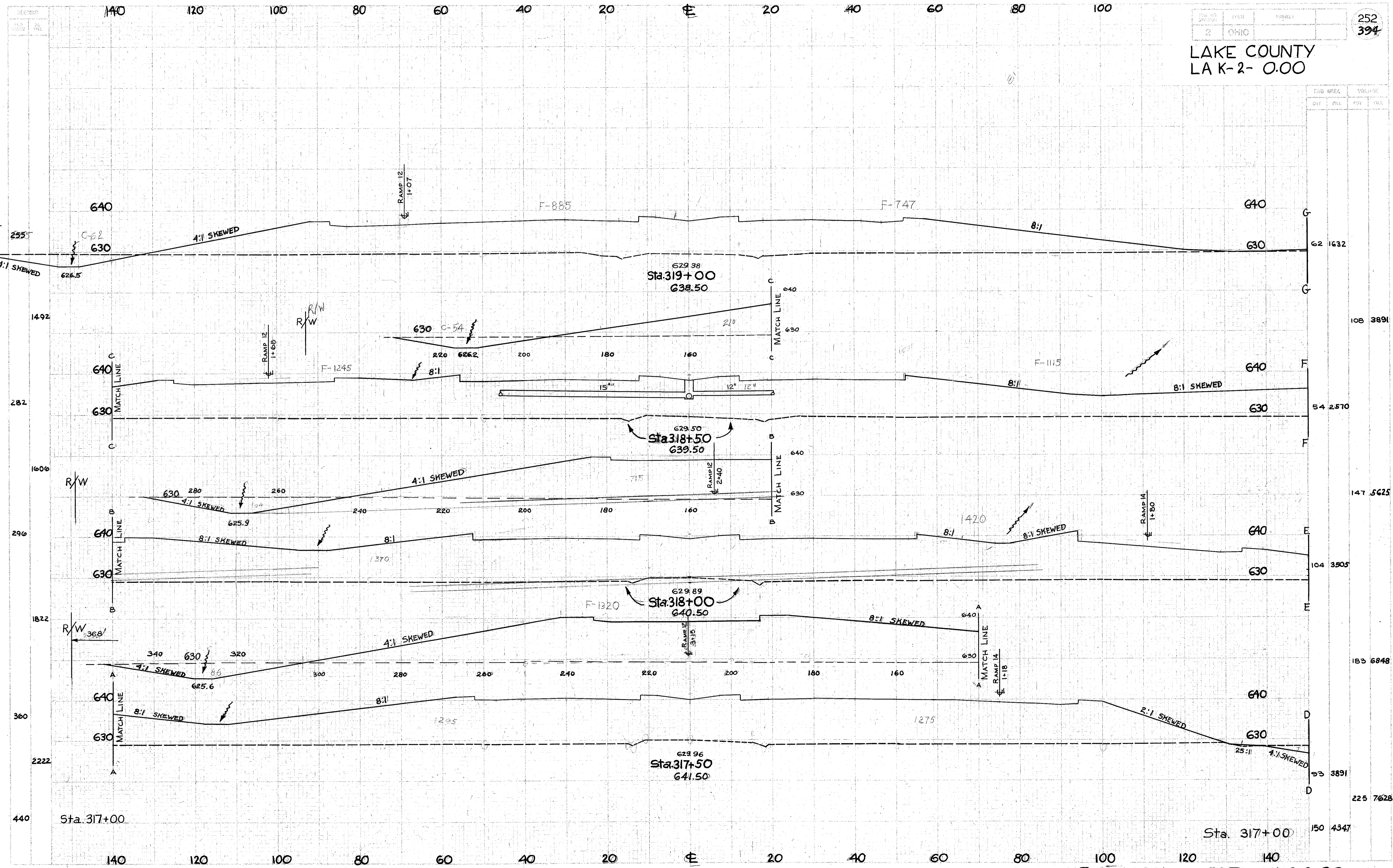
CROSS SECTIONS- STA. 317+50 TO STA. 319+00
