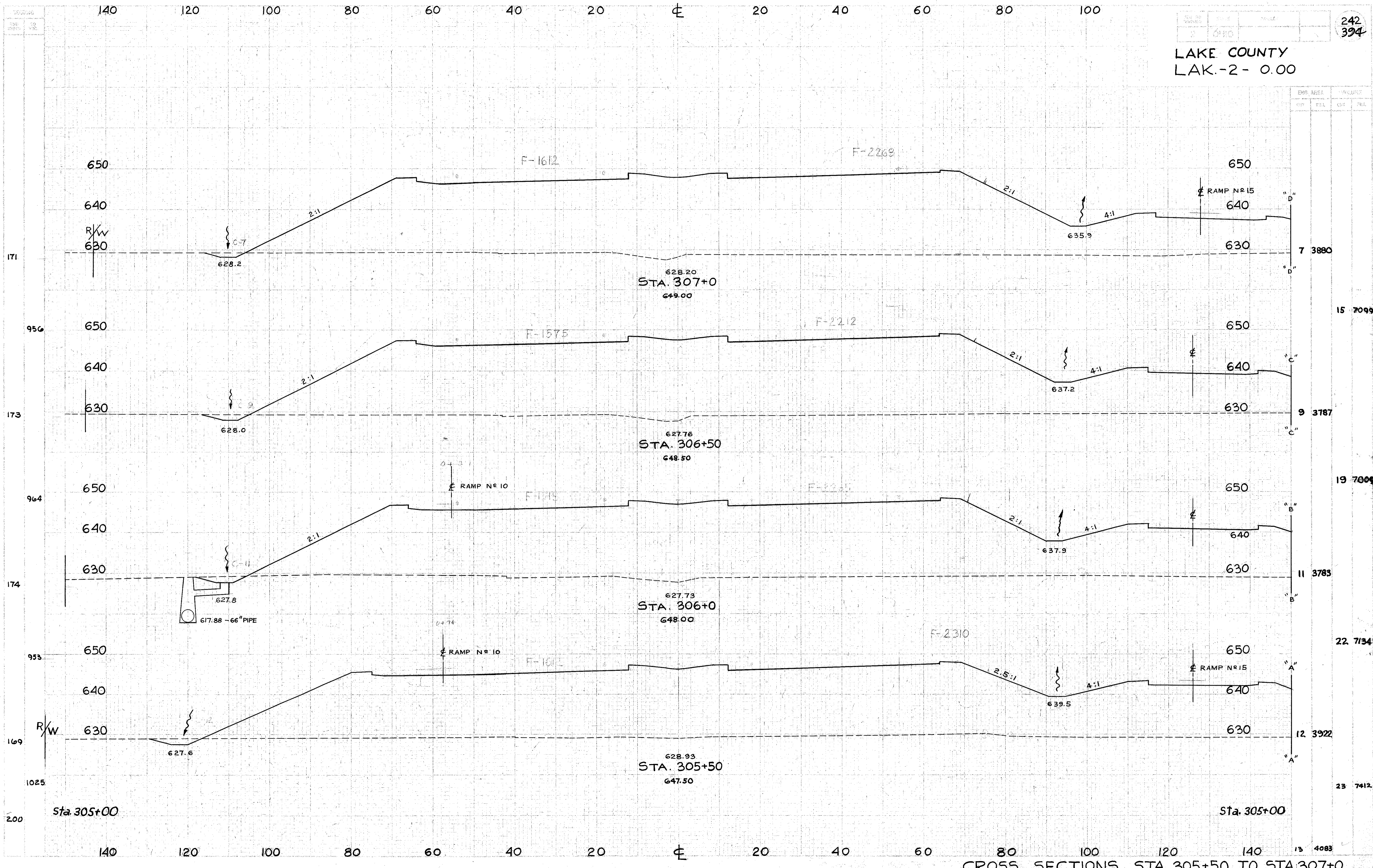
CROSS SECTIONS STA. 305+50 TO STA. 307+0
