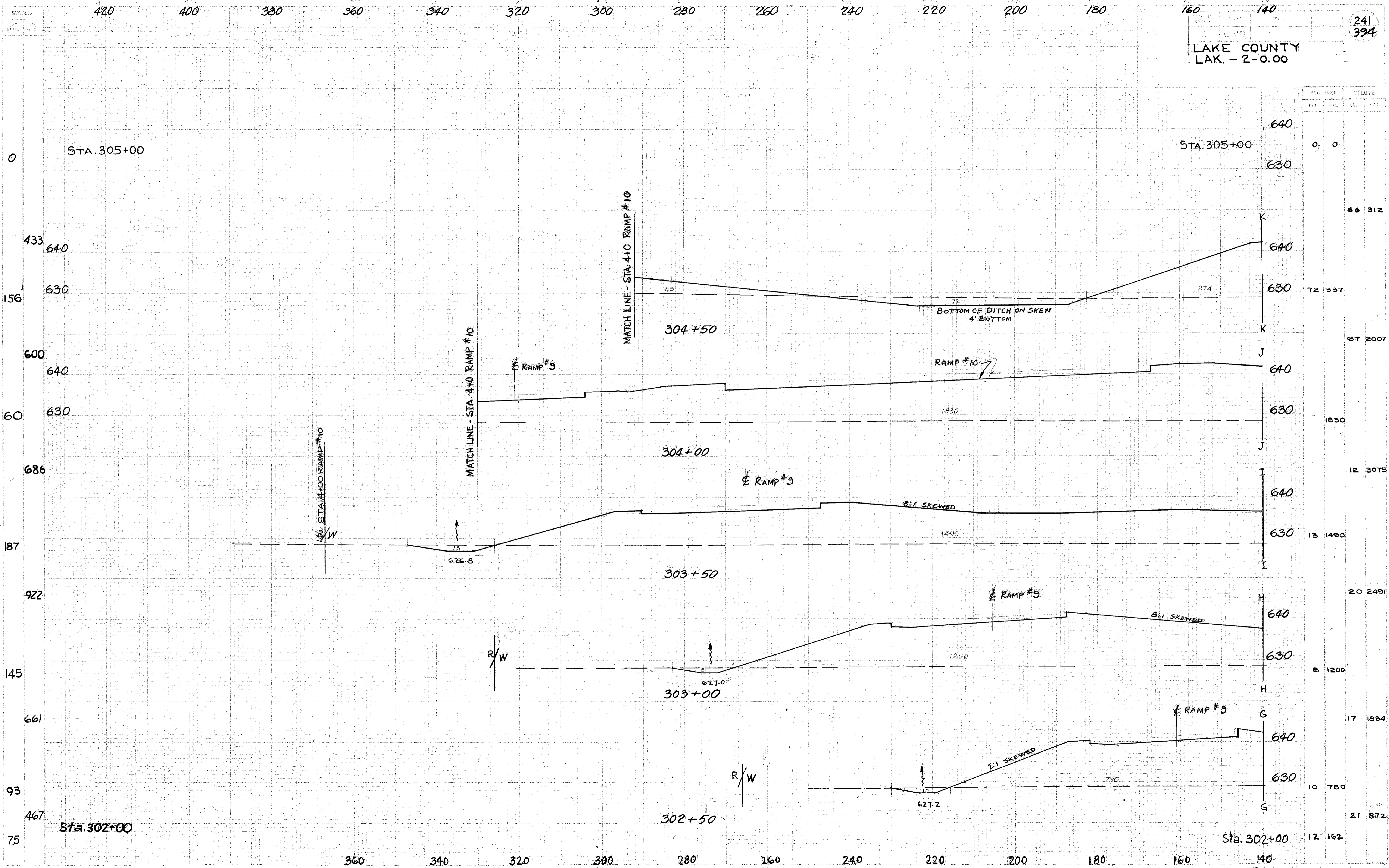
CROSS SECTION EXTENSIONS - STA. 302+50 TO STA. 304+50 - LEFT
