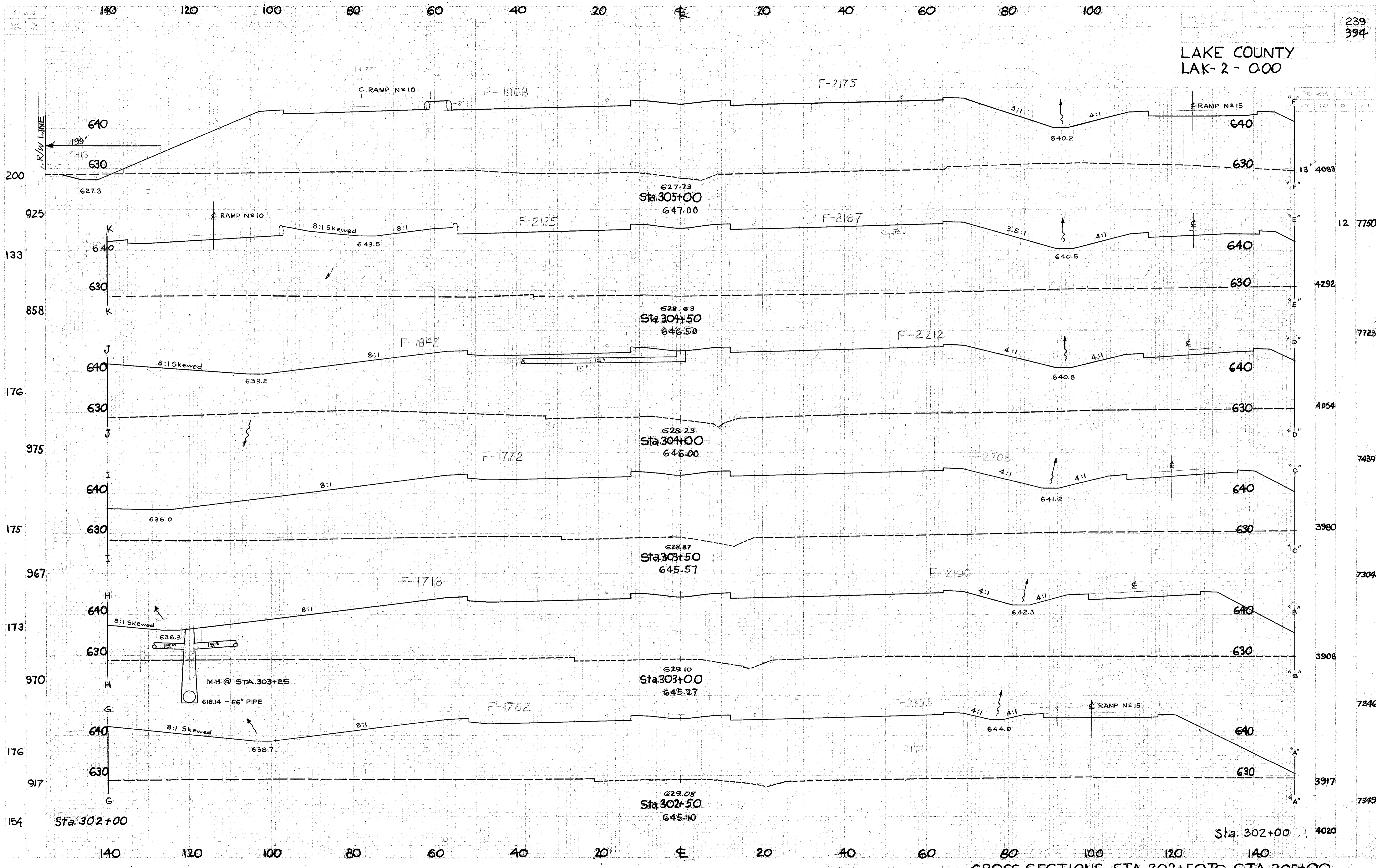
CROSS SECTIONS - STA. 302+50 TO STA. 305+00
