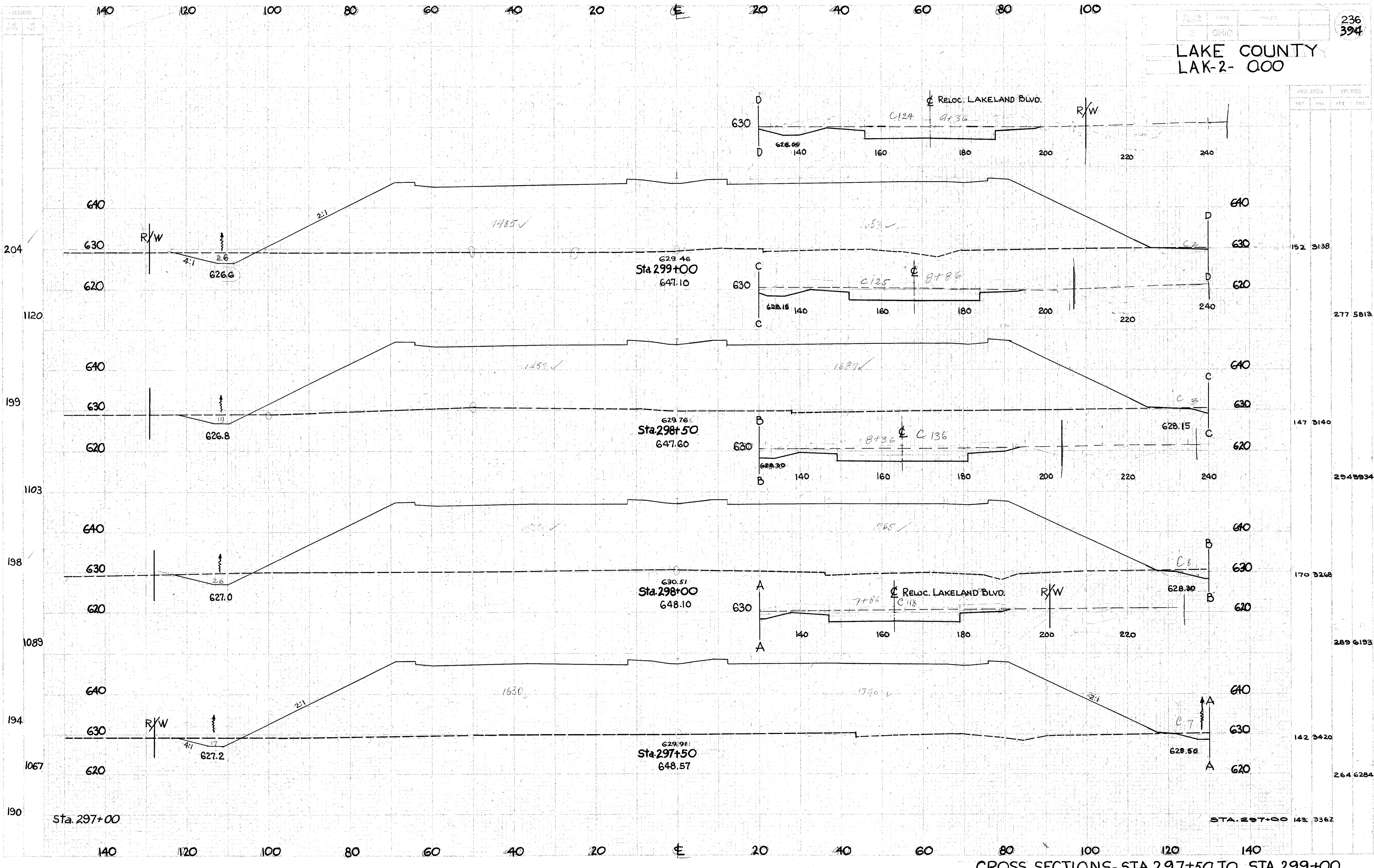
CROSS SECTIONS- STA. 297+50 TO STA. 299+00
