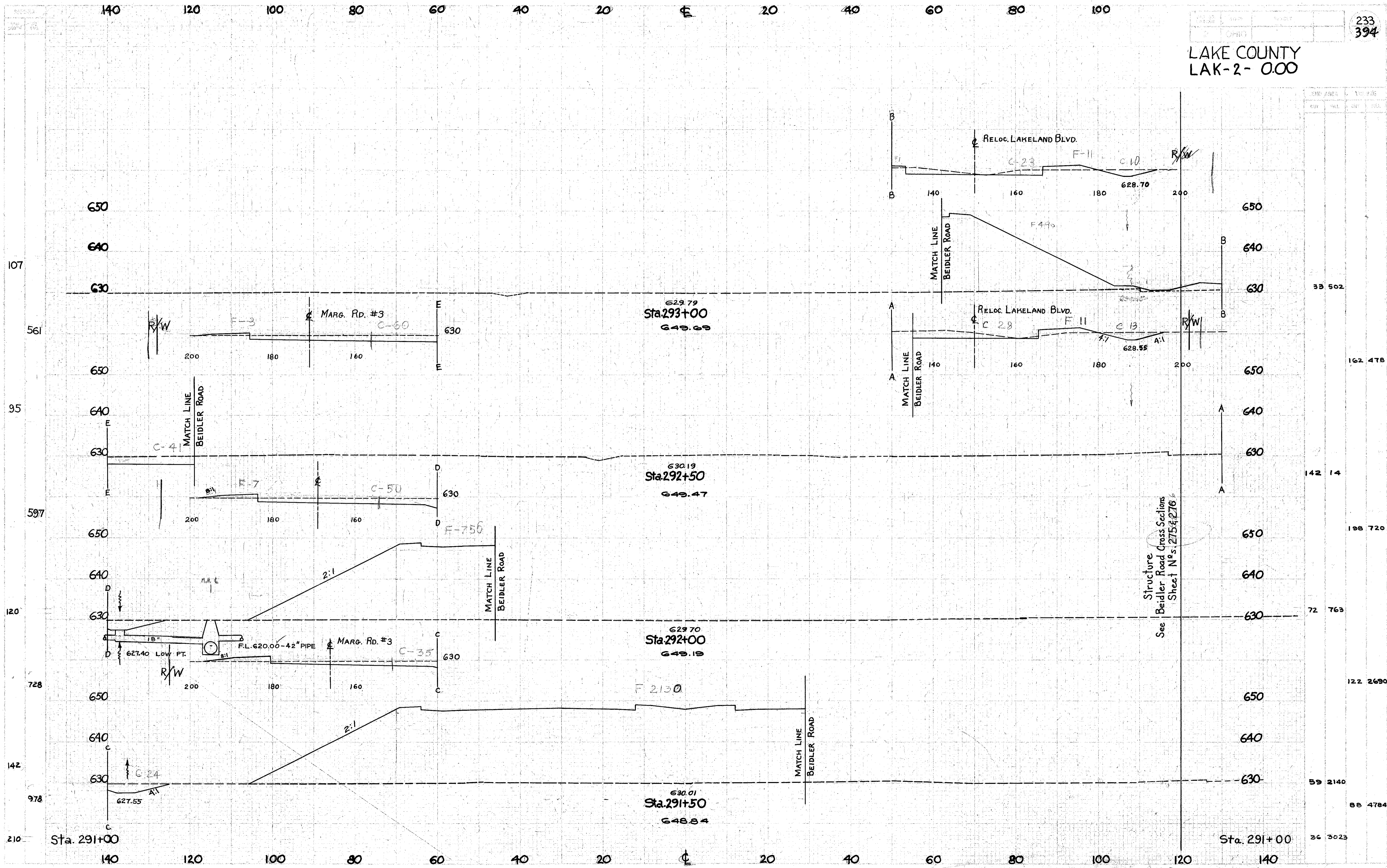
CROSS SECTIONS- STA. 291+50 TO STA. 293+00
