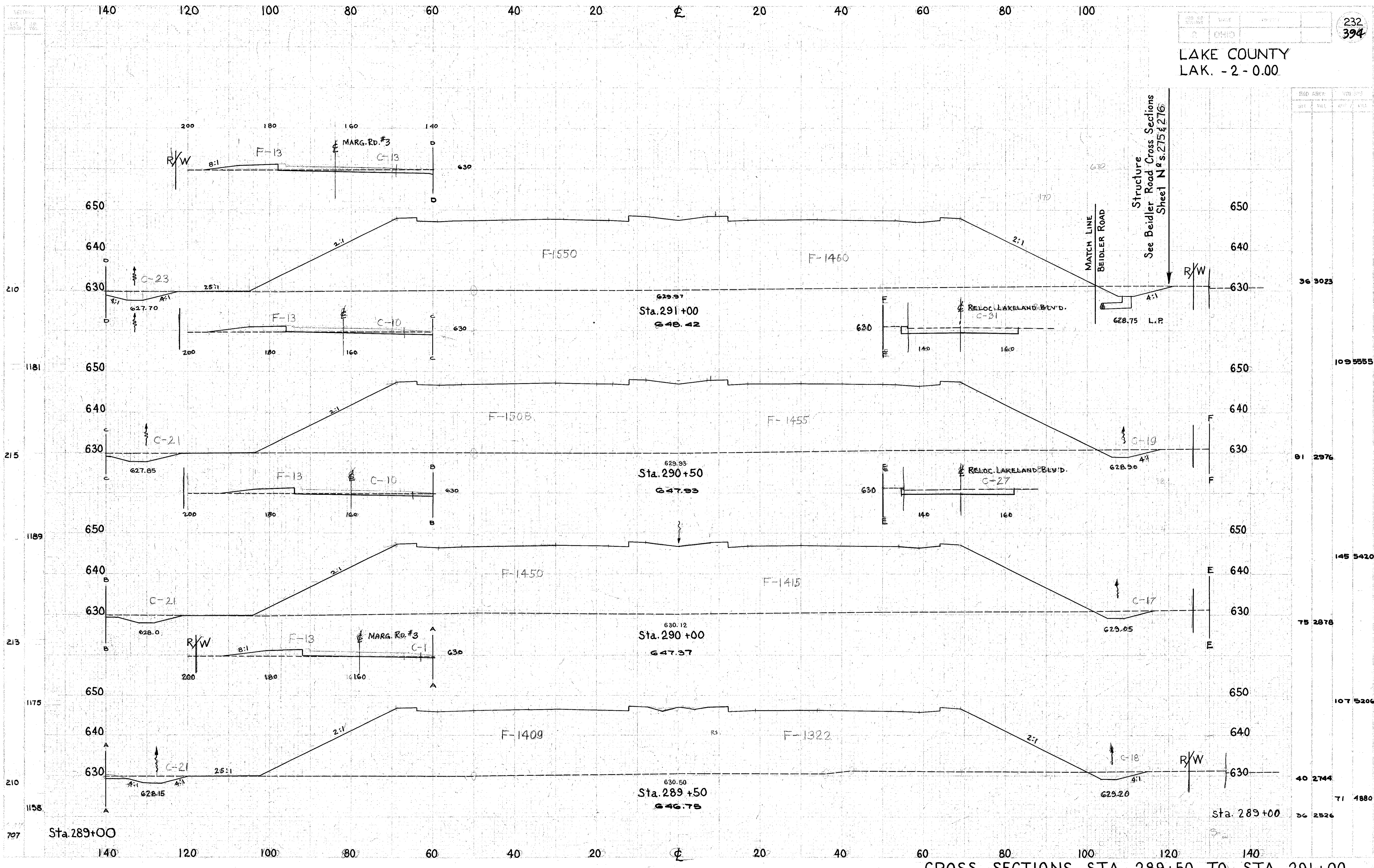
CROSS SECTIONS STA. 289+50 TO STA. 291+00
