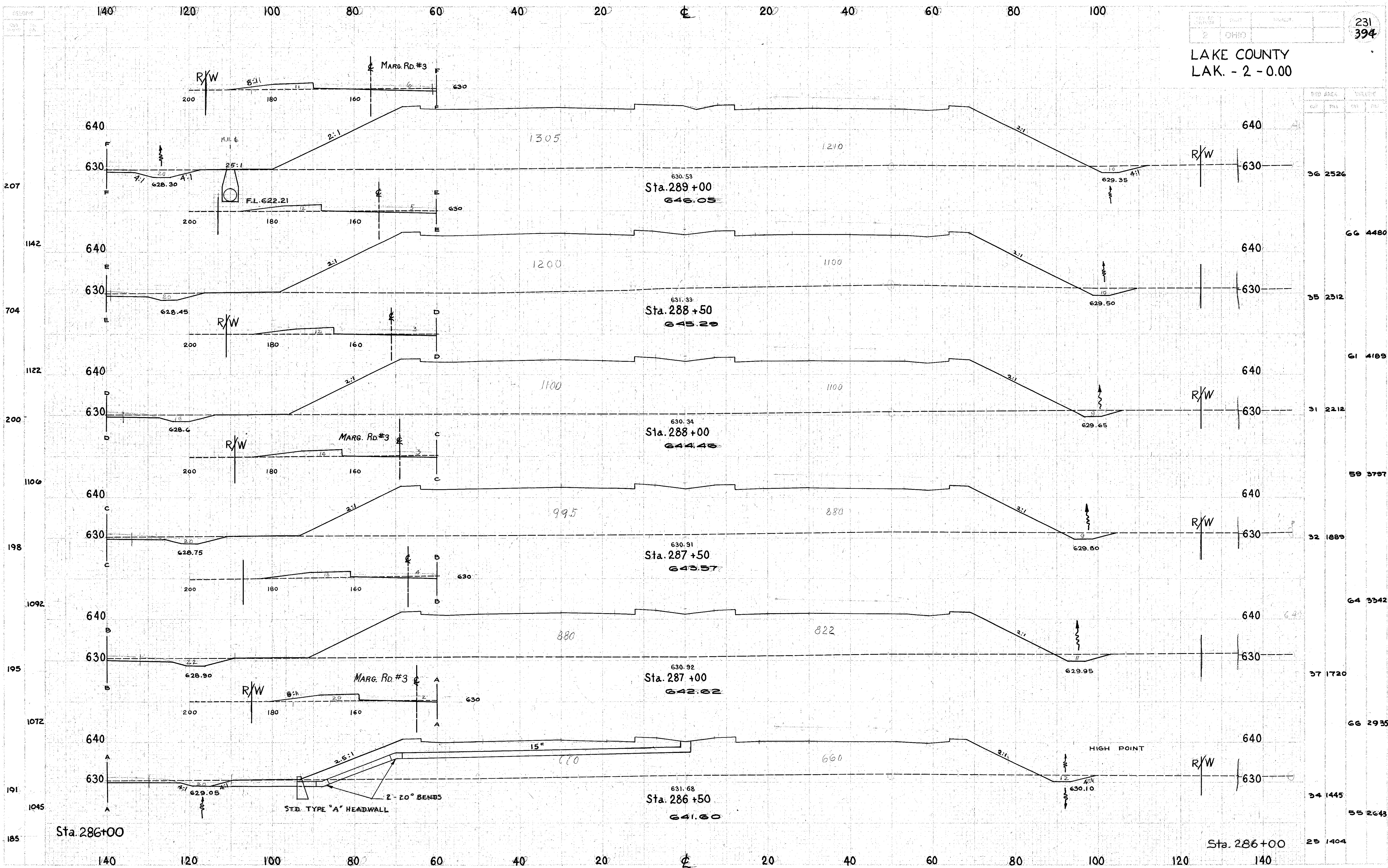
CROSS SECTIONS STA. 286+50 TO STA. 289+00
