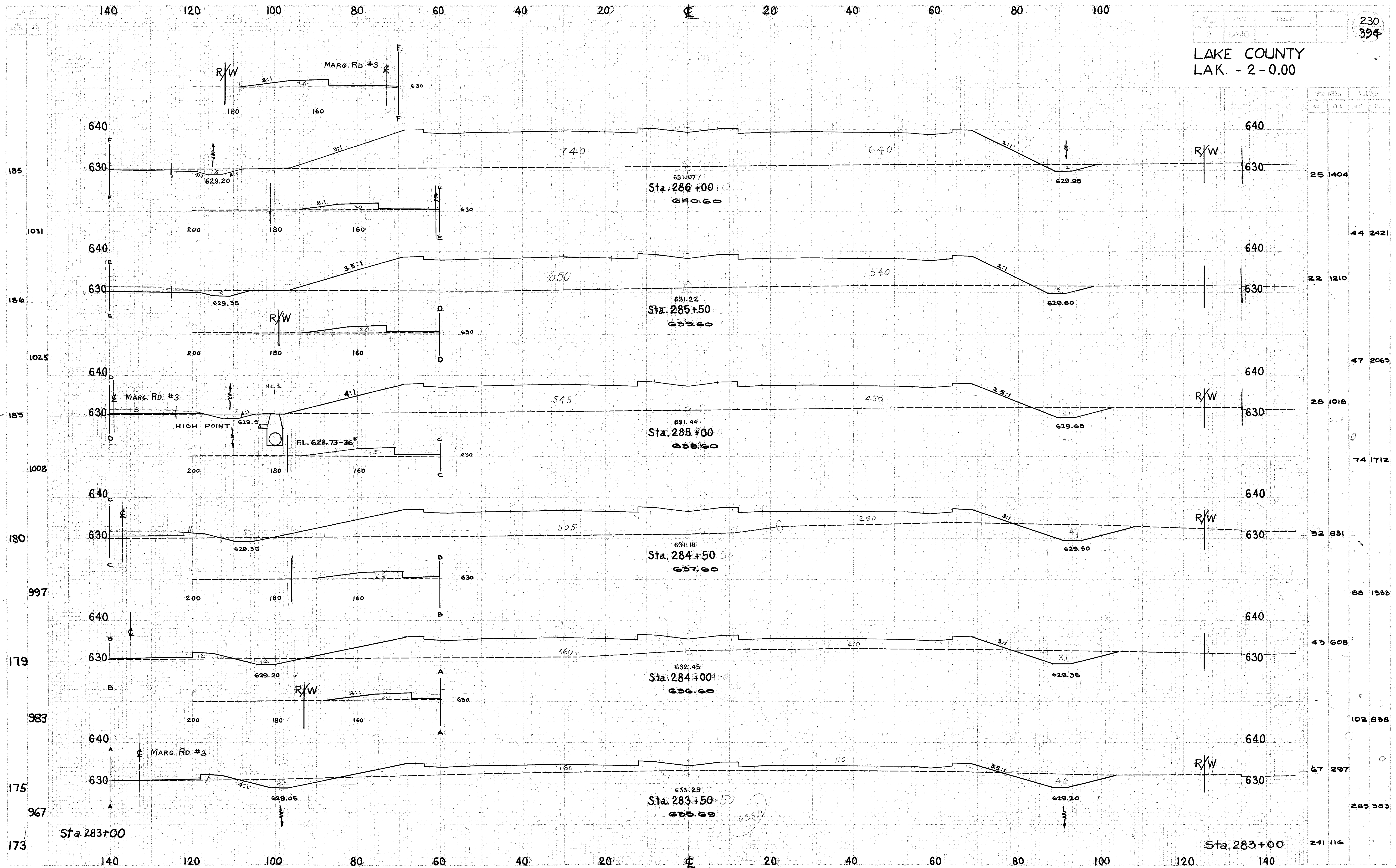
CROSS SECTIONS STA. 283+50 TO STA. 286+00
