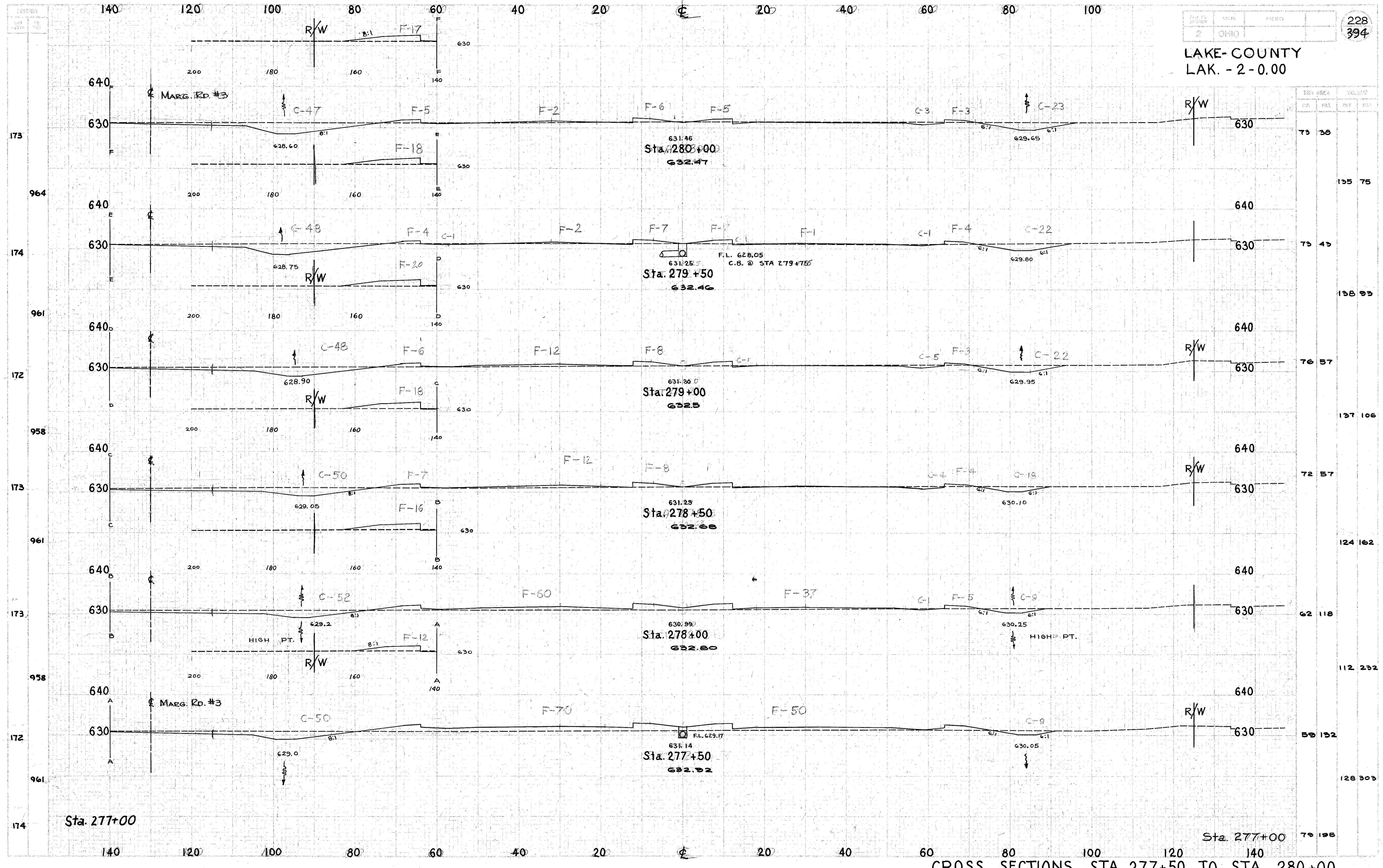
CROSS SECTIONS STA. 277+50 TO STA. 280+00
