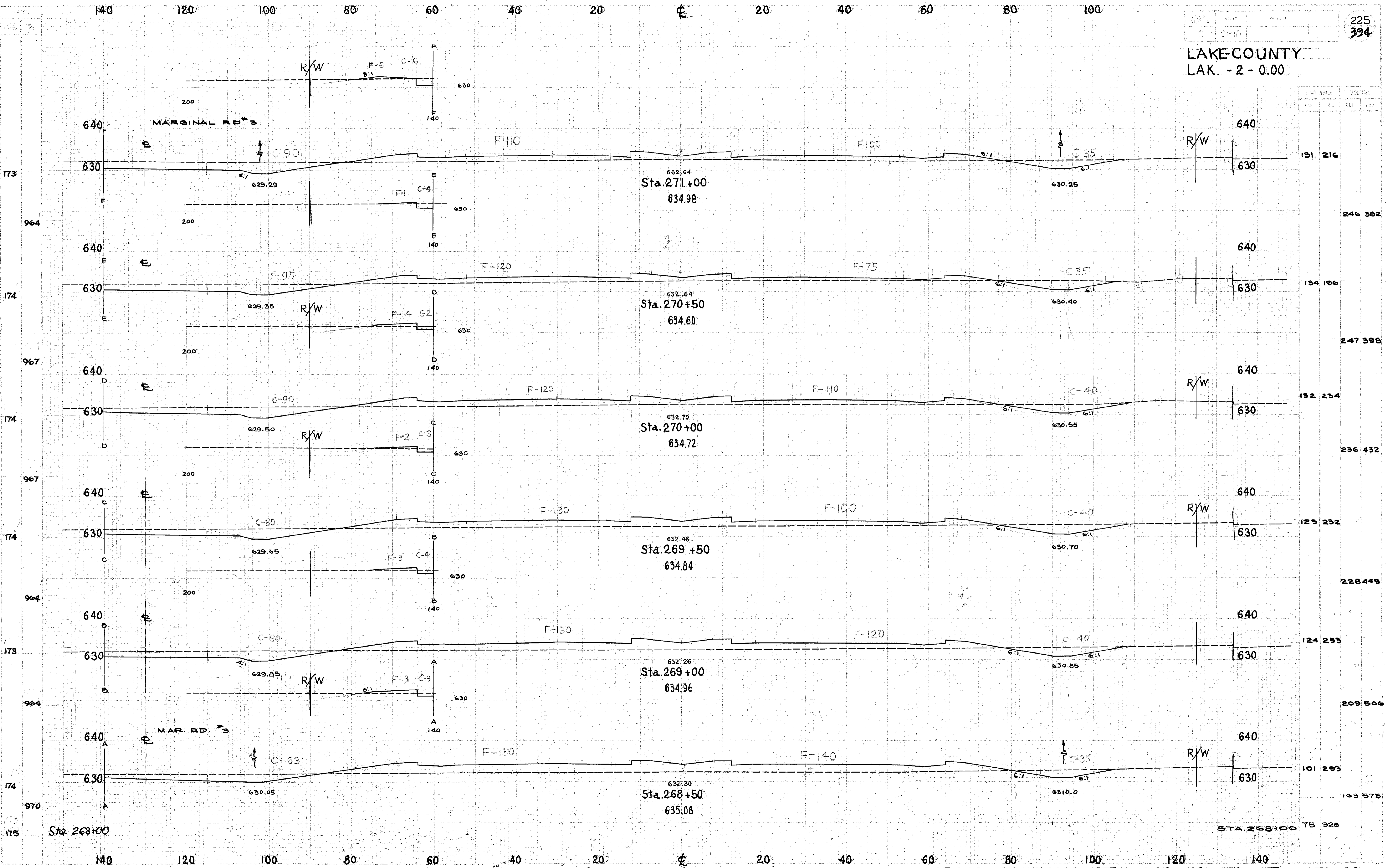
CROSS SECTIONS STA. 268+50 TO STA. 271+00
