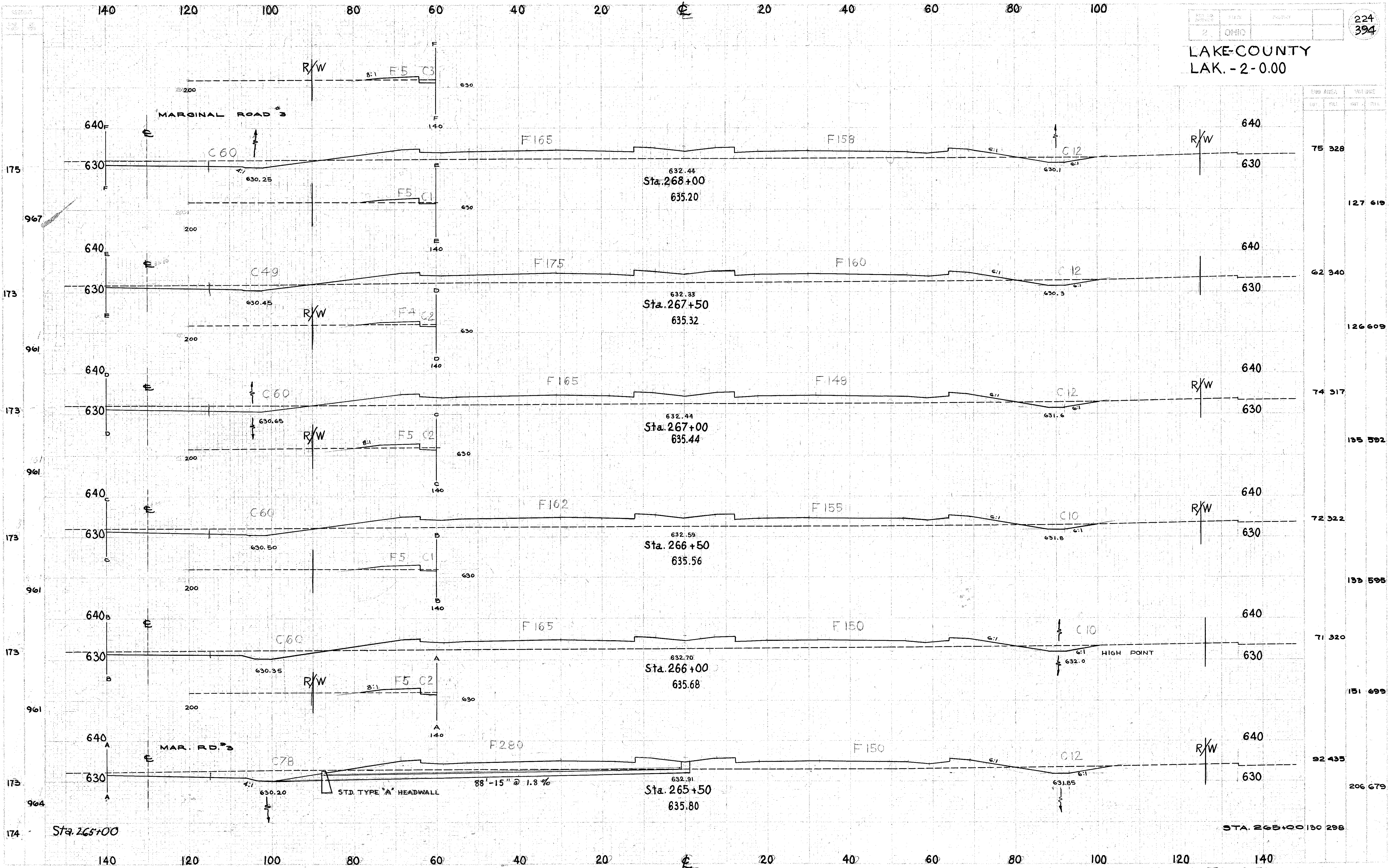
CROSS SECTIONS STA. 265+50 TO STA. 268+00
