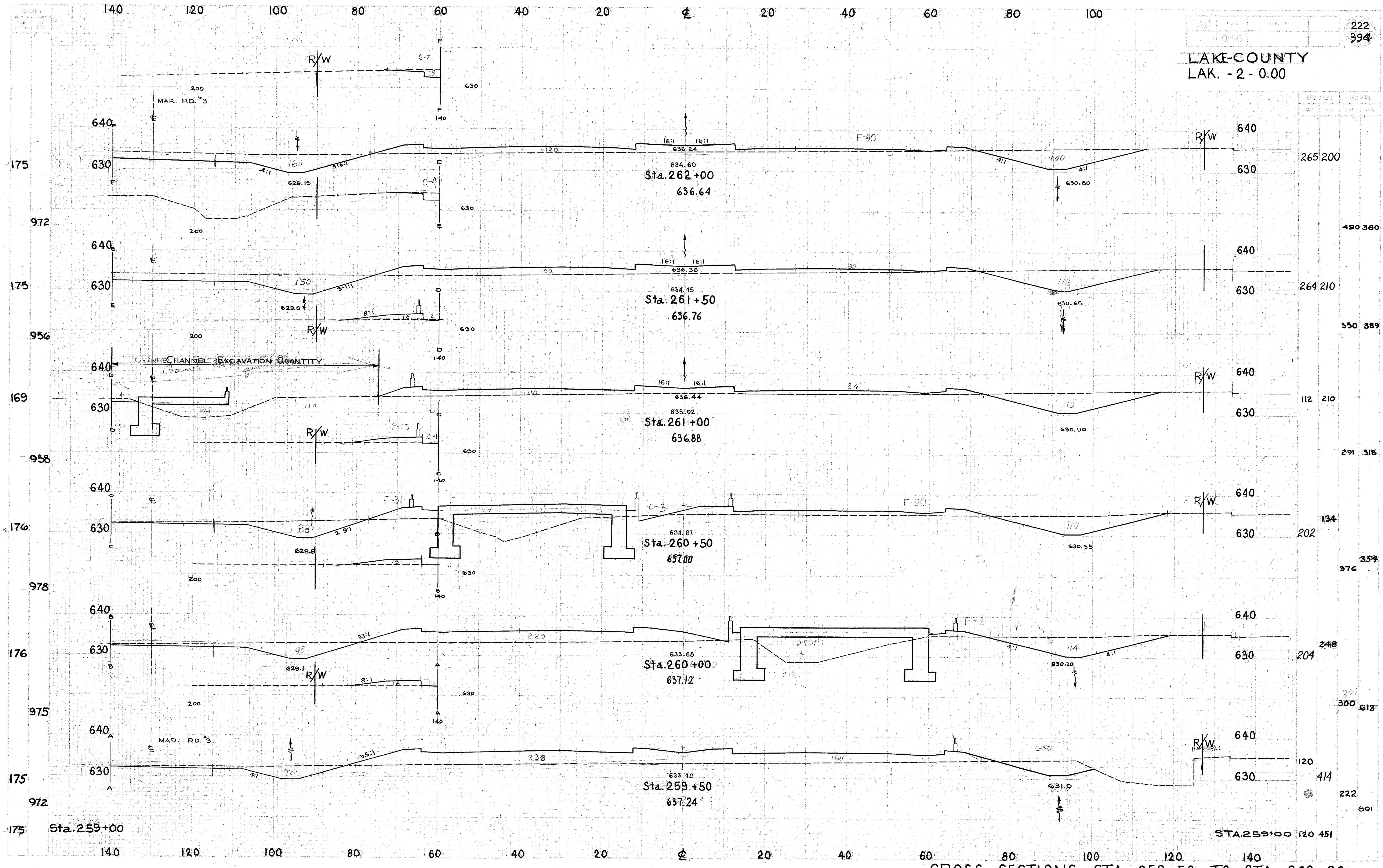
CROSS SECTIONS STA. 259+50 TO STA. 262+00
