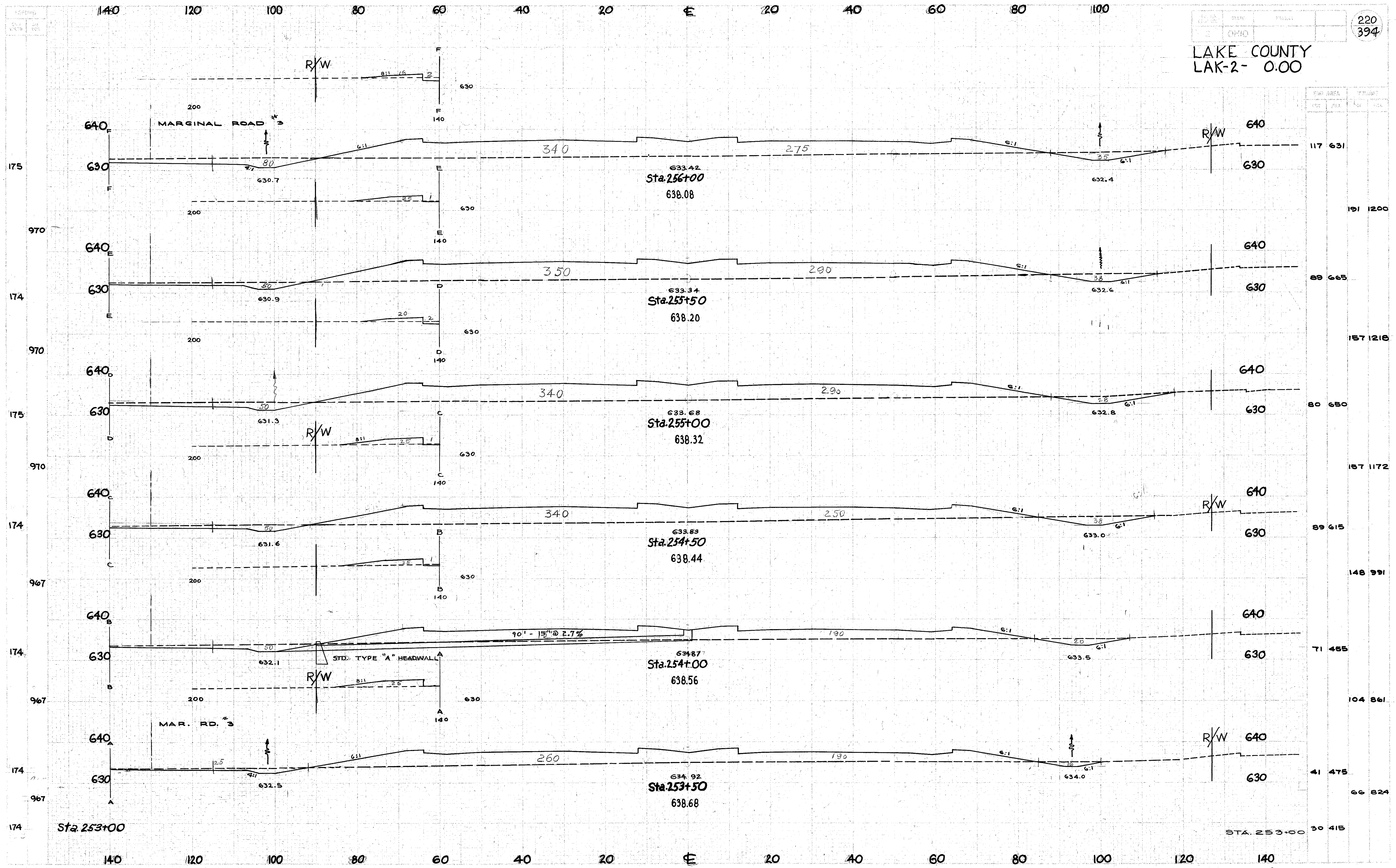
CROSS SECTIONS- STA. 253+50 TO STA. 256+00
