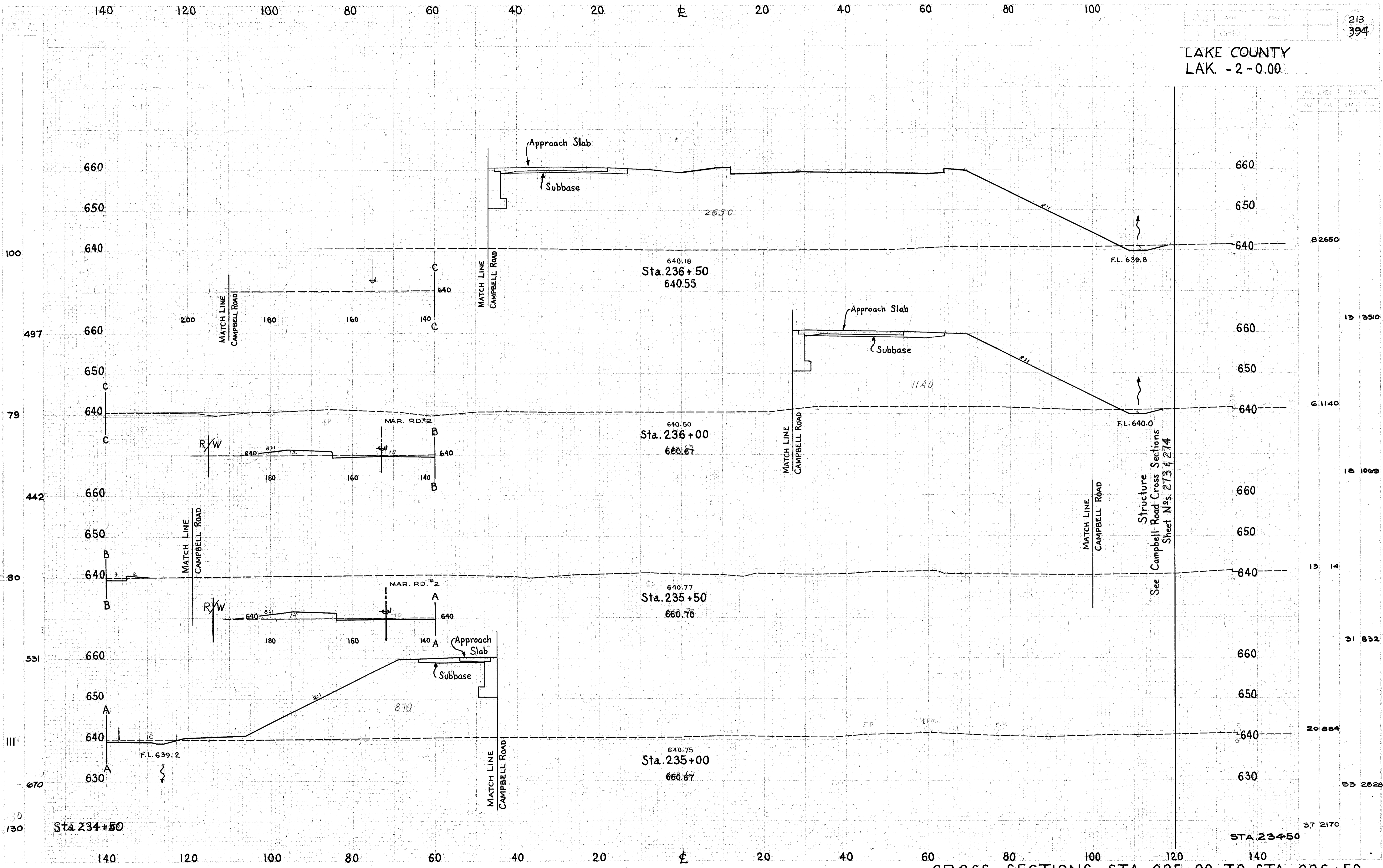
CROSS SECTIONS STA. 235+00 TO STA. 236+50
