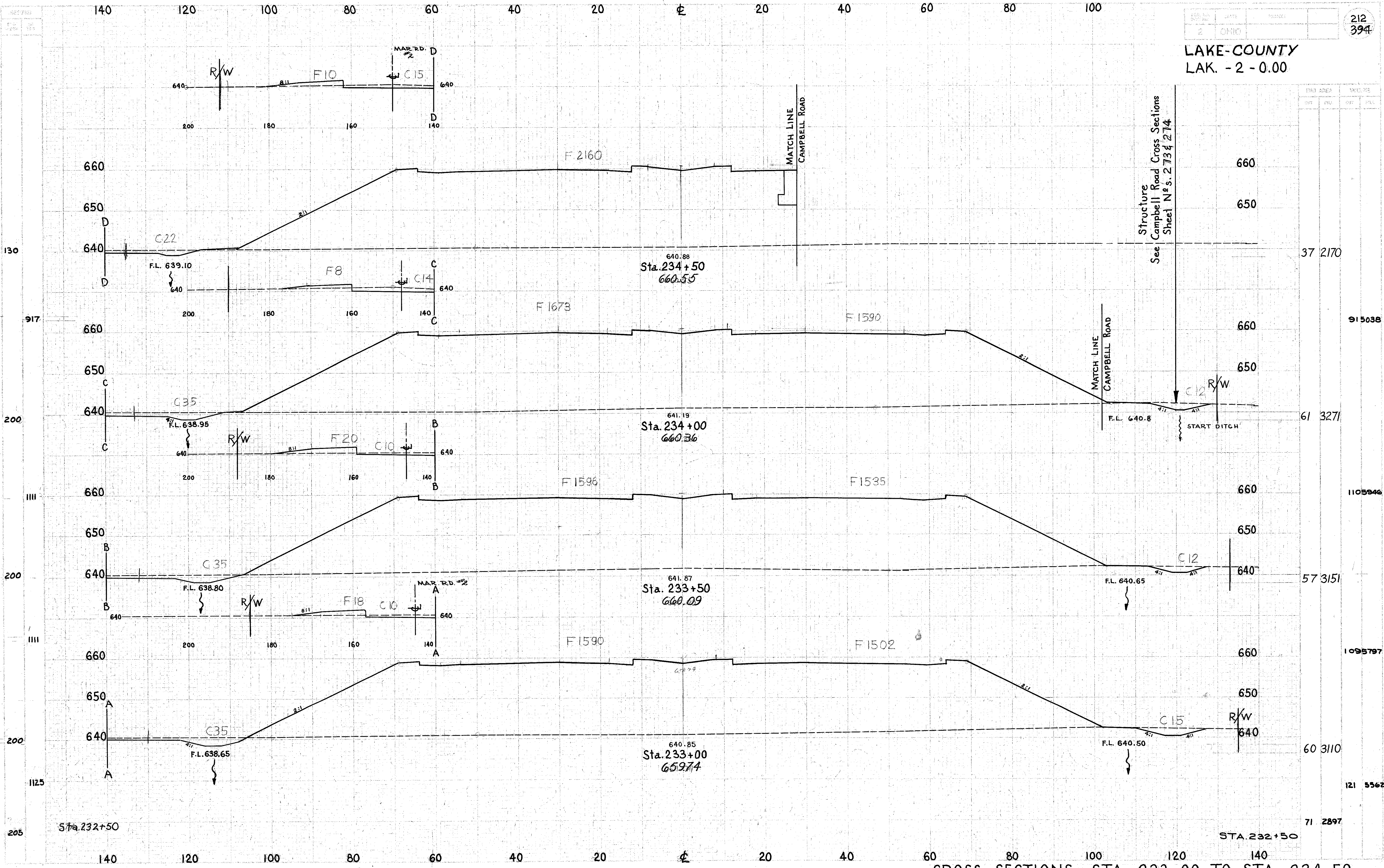
CROSS SECTIONS STA. 233+00 TO STA. 234+50
