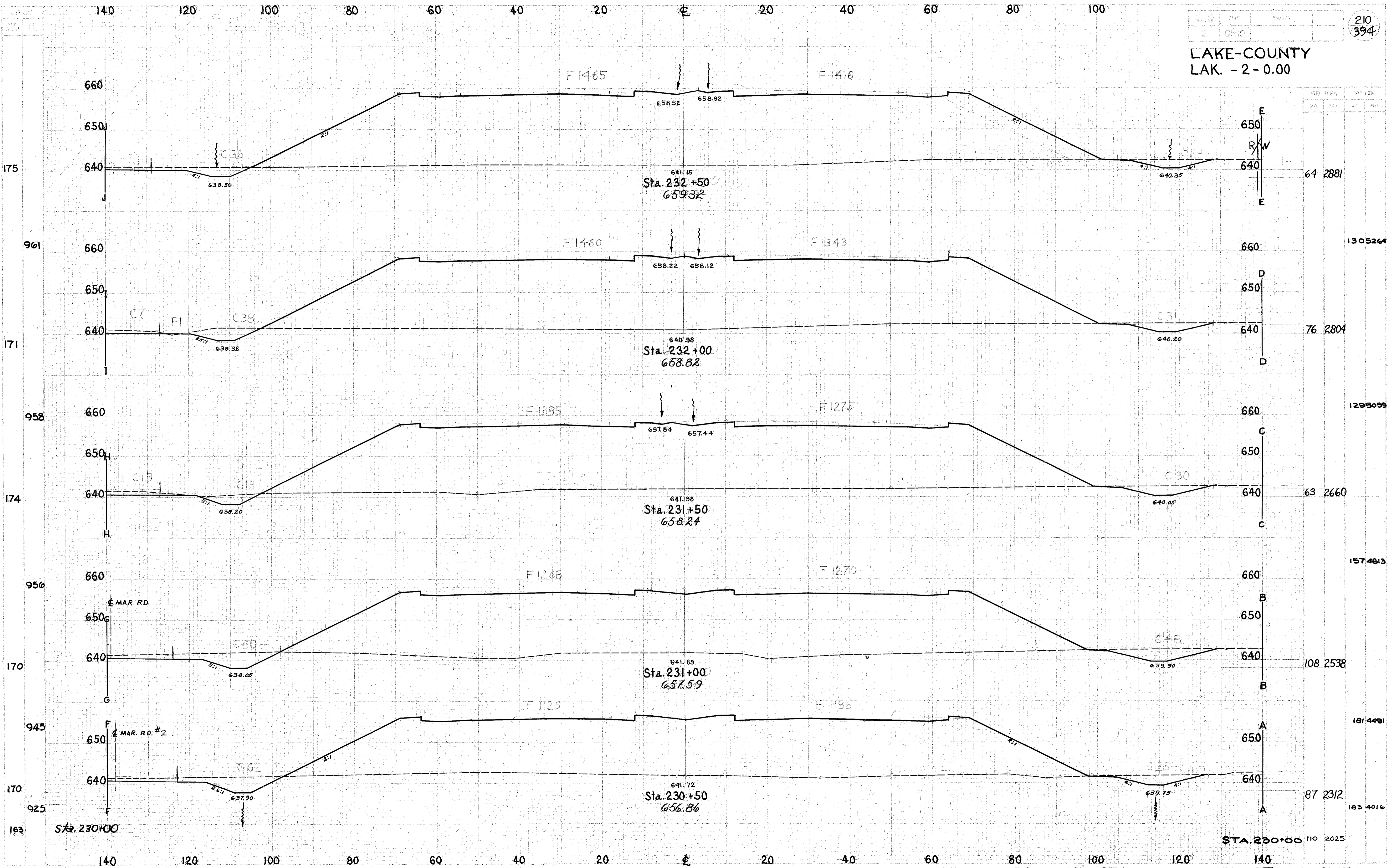
CROSS SECTIONS STA. 230+50 TO STA. 232+50
