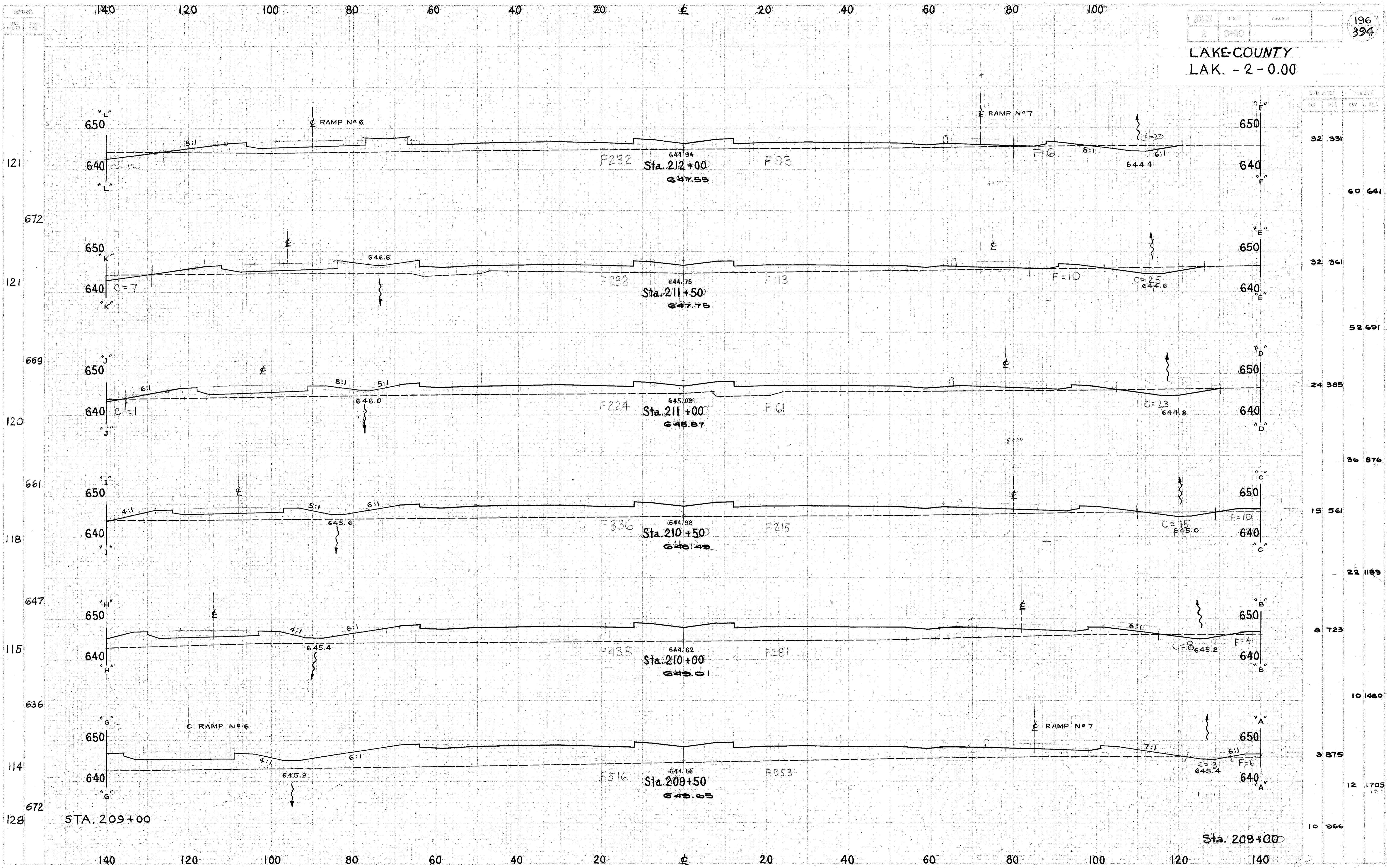
CROSS SECTIONS STA. 209+50 TO STA. 212+00
