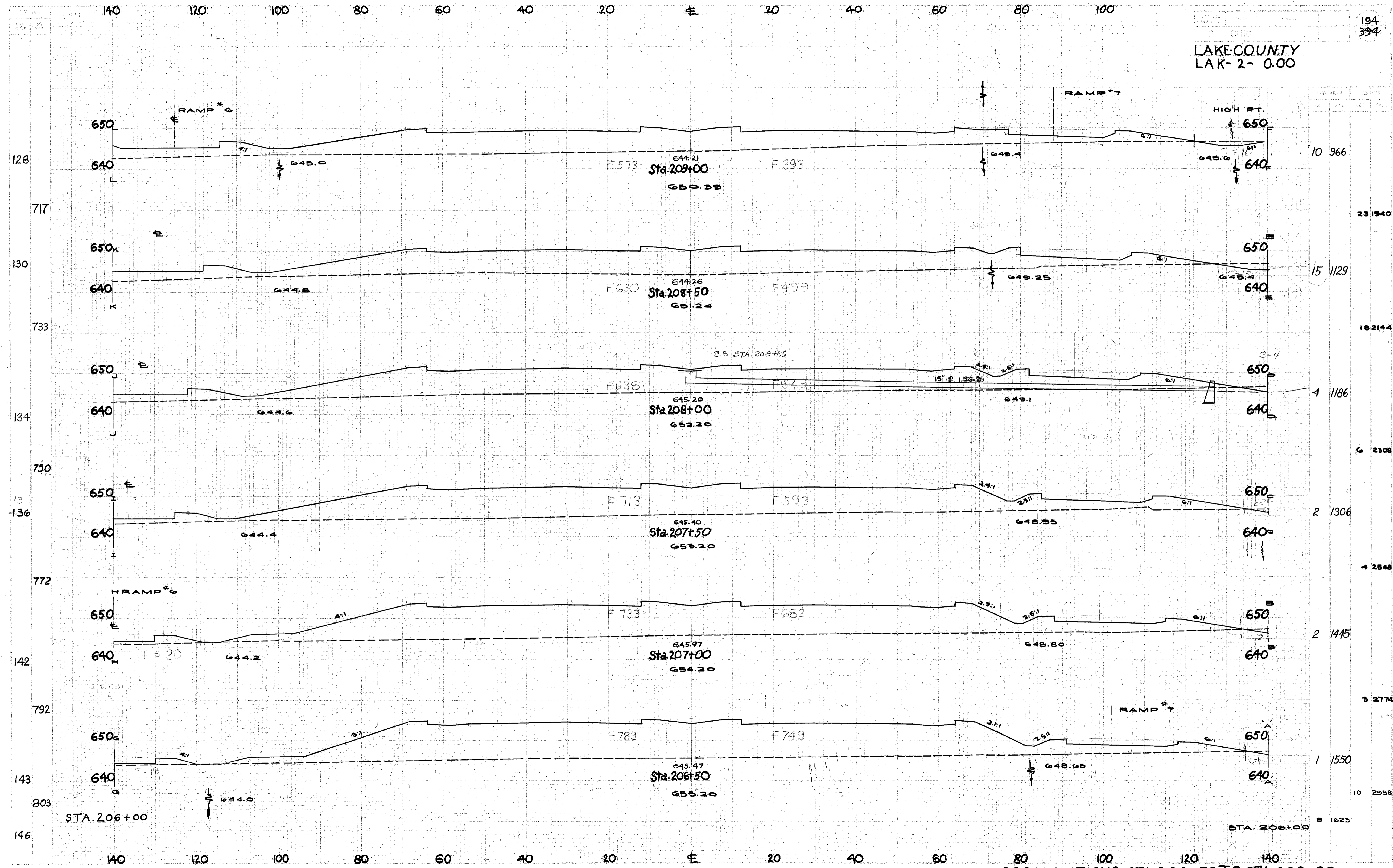
CROSS SECTIONS-STA. 206+50 TO STA. 209+00
