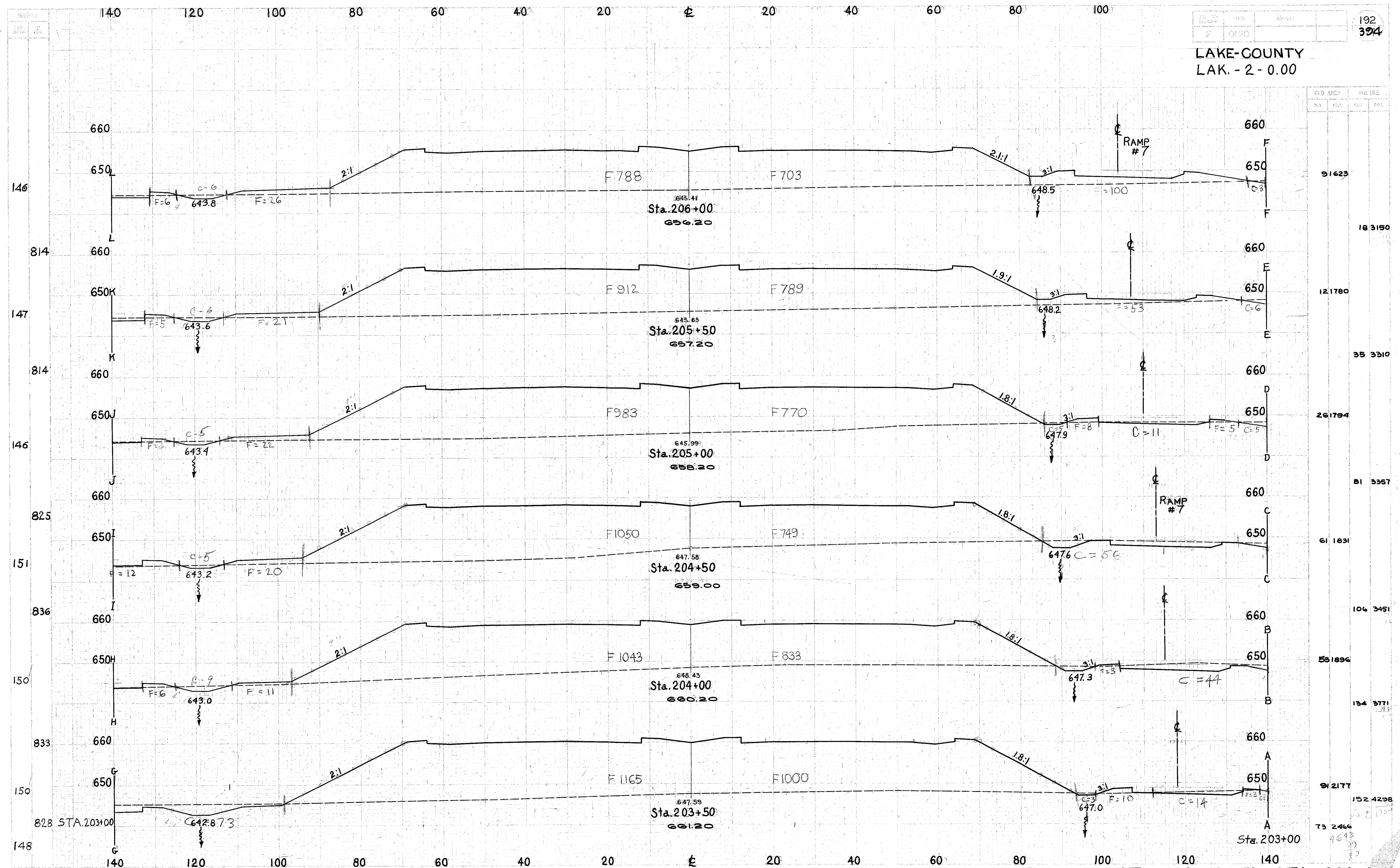
CROSS SECTIONS STA. 203+50 TO STA. 206+00
