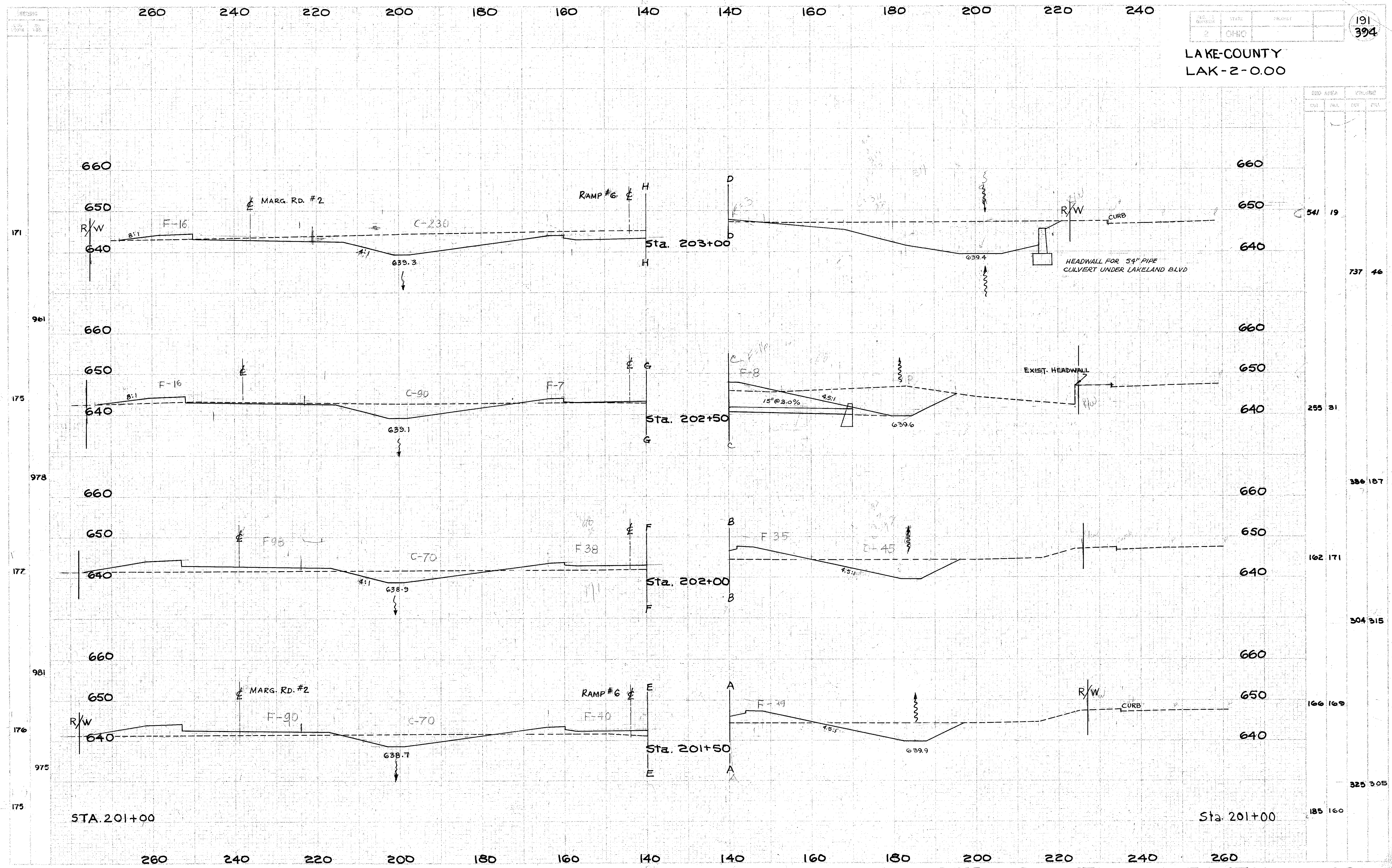
CROSS SECTION EXTENSIONS STA. 201+50 TO STA. 203+00
