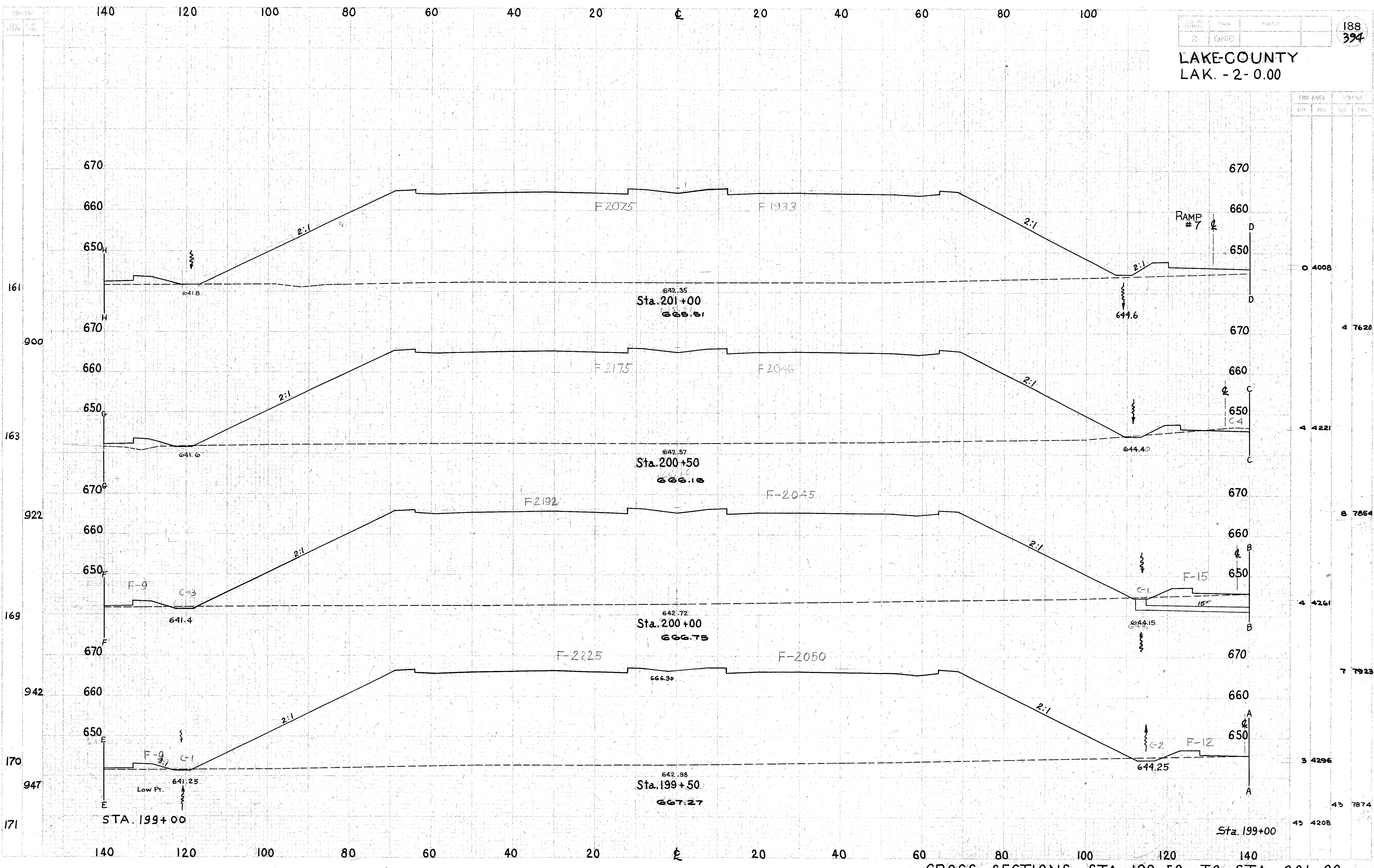
CROSS SECTIONS STA. 199+50 TO STA. 201+00
