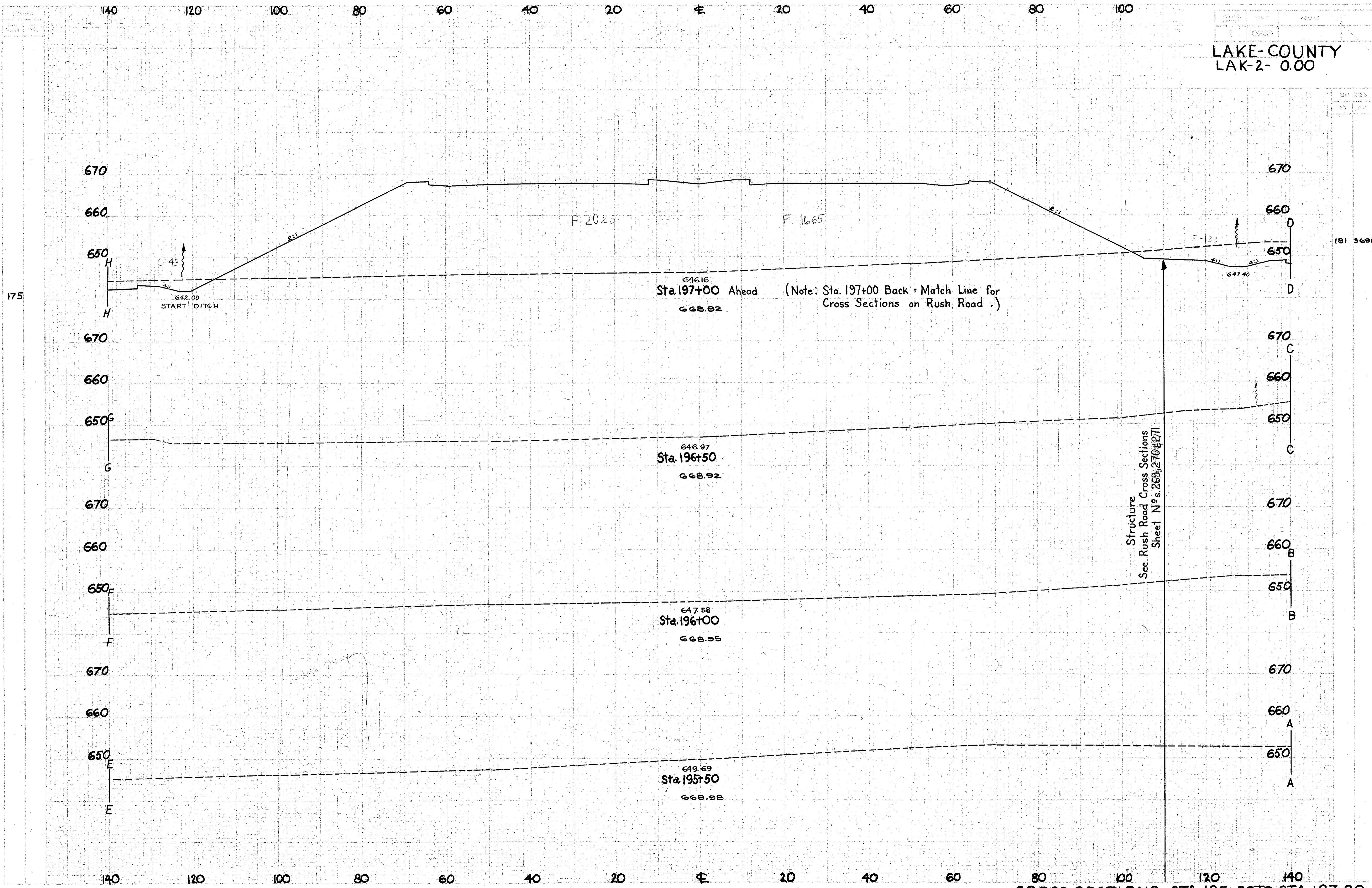
CROSS SECTIONS - STA. 195+50 TO STA. 197+00
