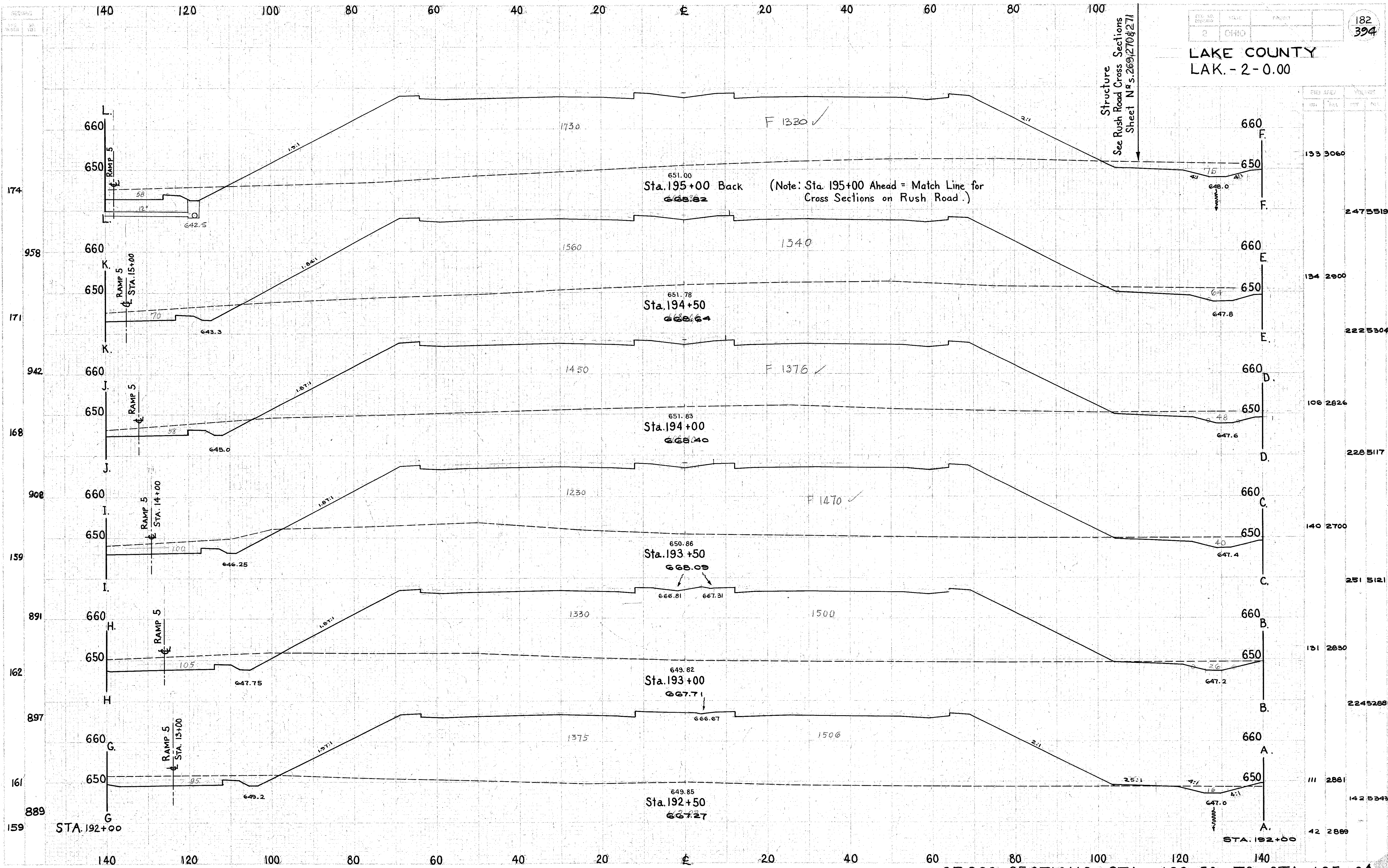
CROSS SECTIONS STA. 192+50 TO STA. 195+00
