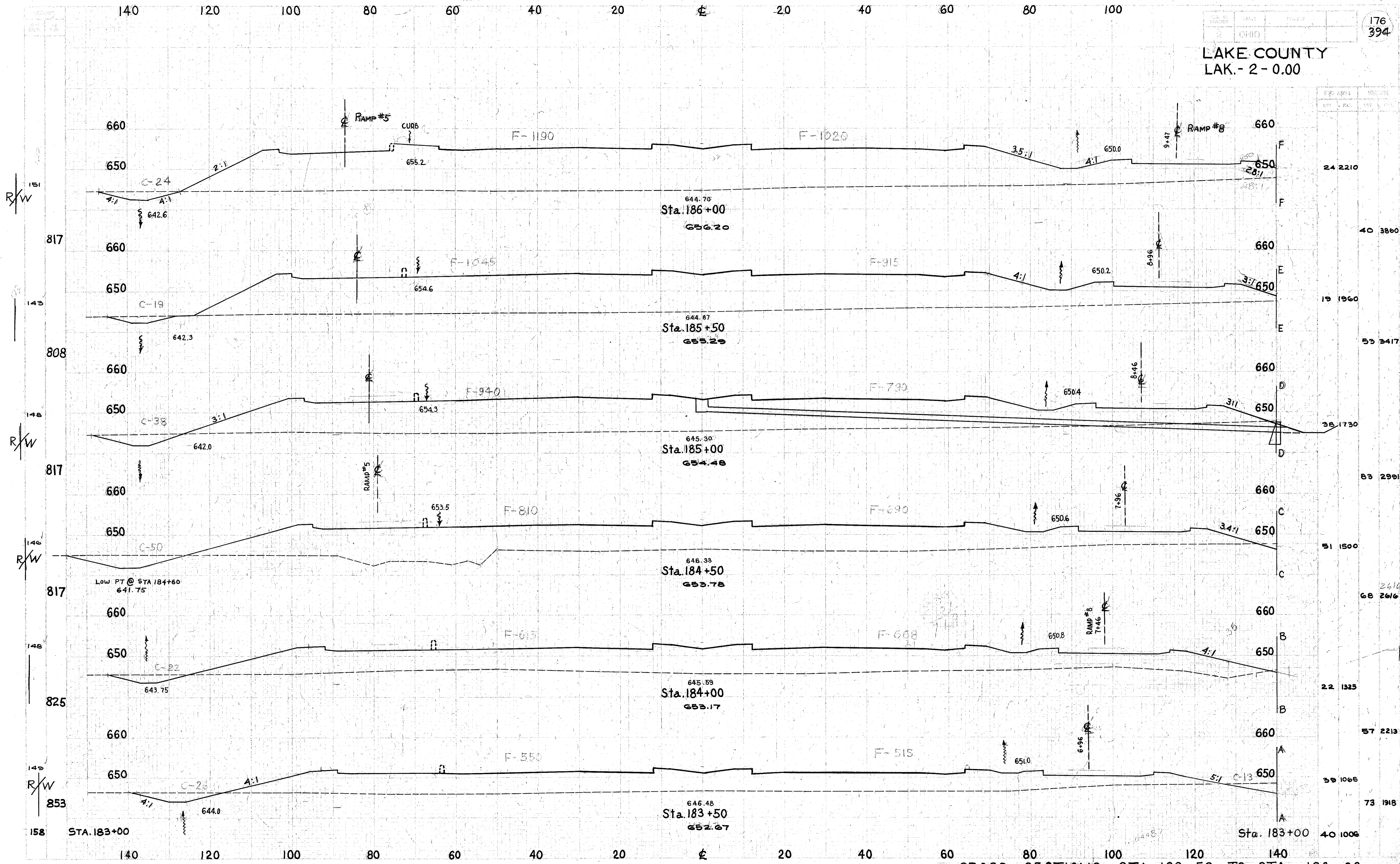
CROSS SECTIONS STA. 183+50 TO STA. 186+00
