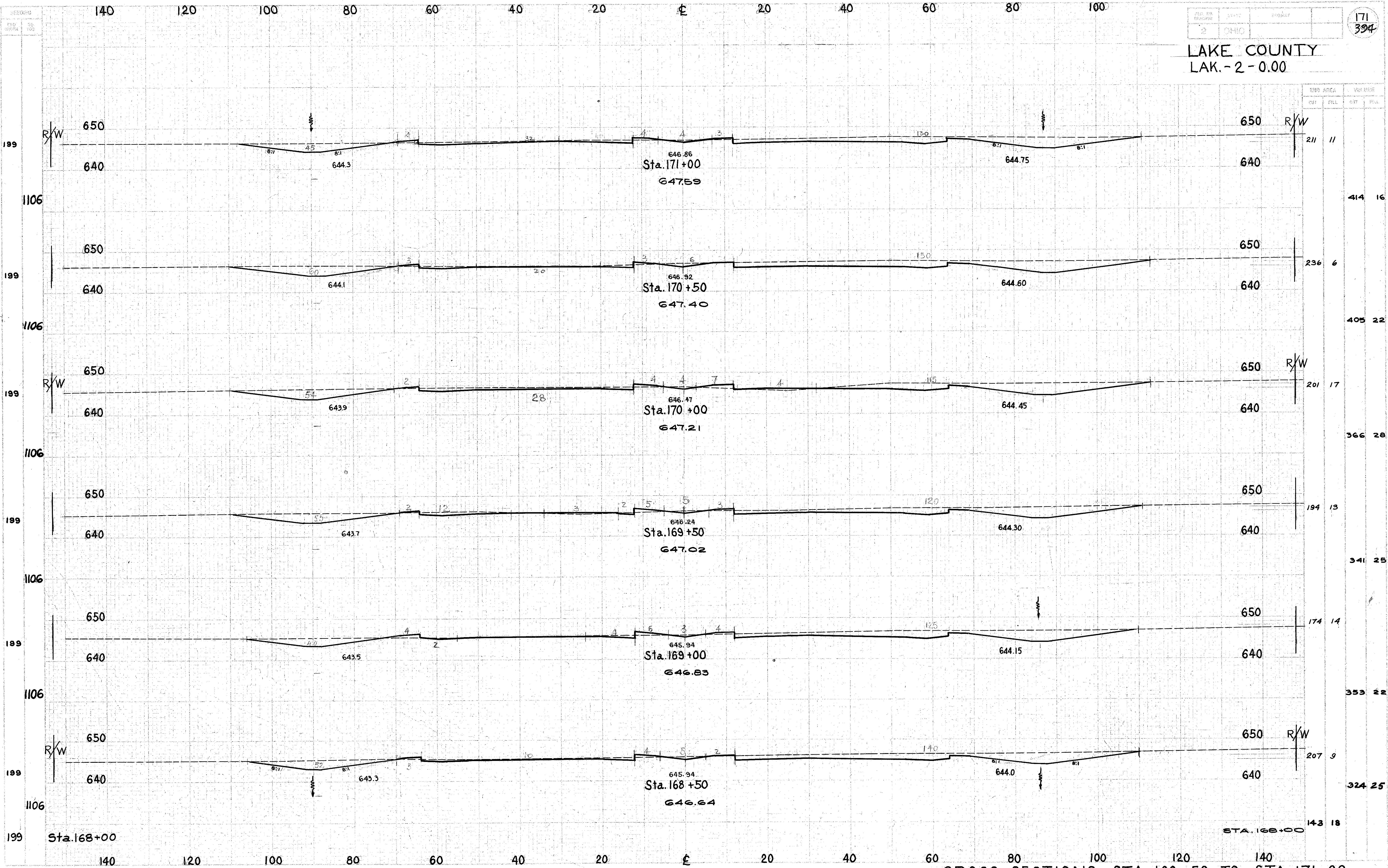
CROSS SECTIONS STA. 168+50 TO STA. 171+00
