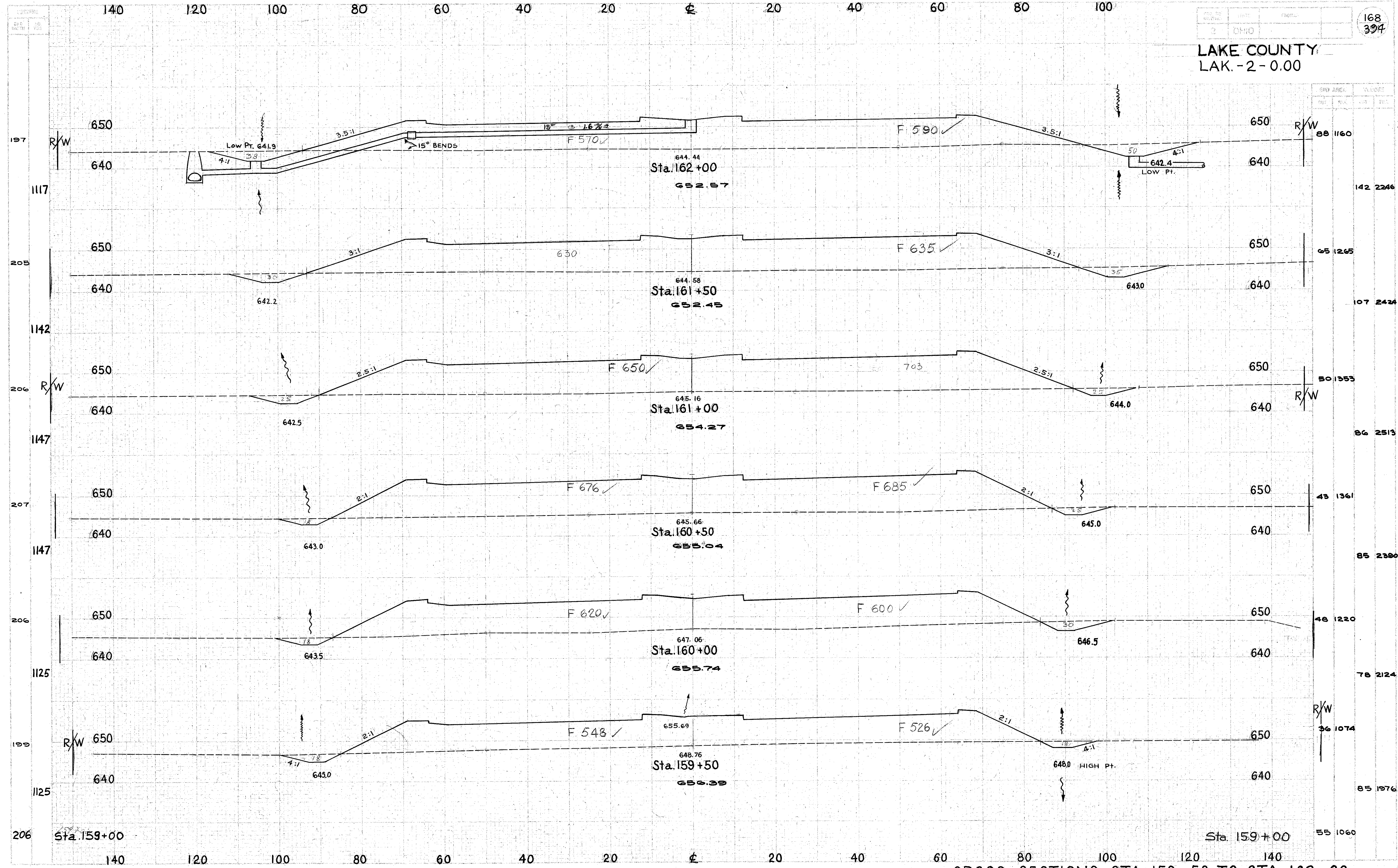
CROSS SECTIONS STA. 159+50 TO STA. 162+00
