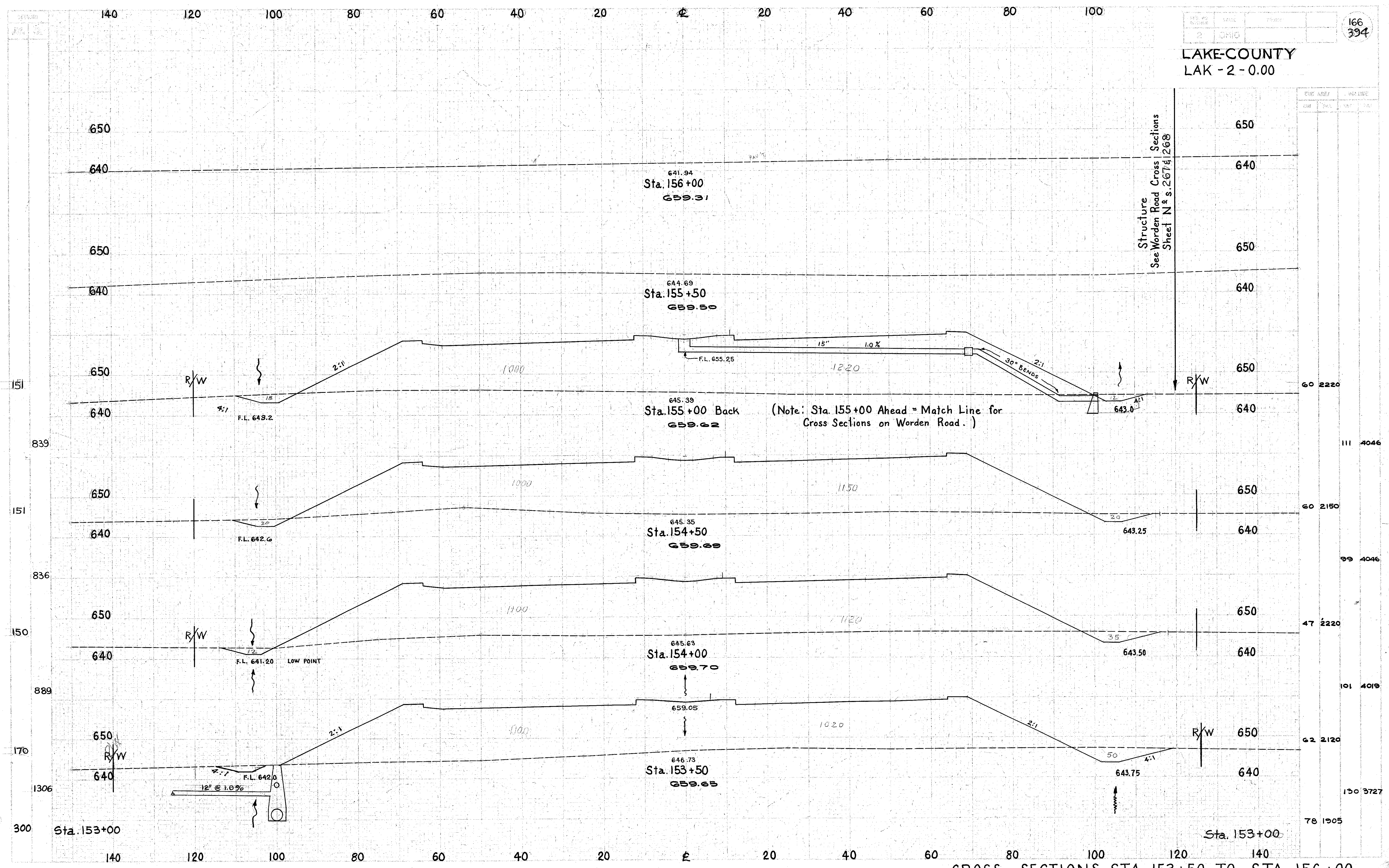
CROSS SECTIONS STA. 153+50 TO STA. 156+00
