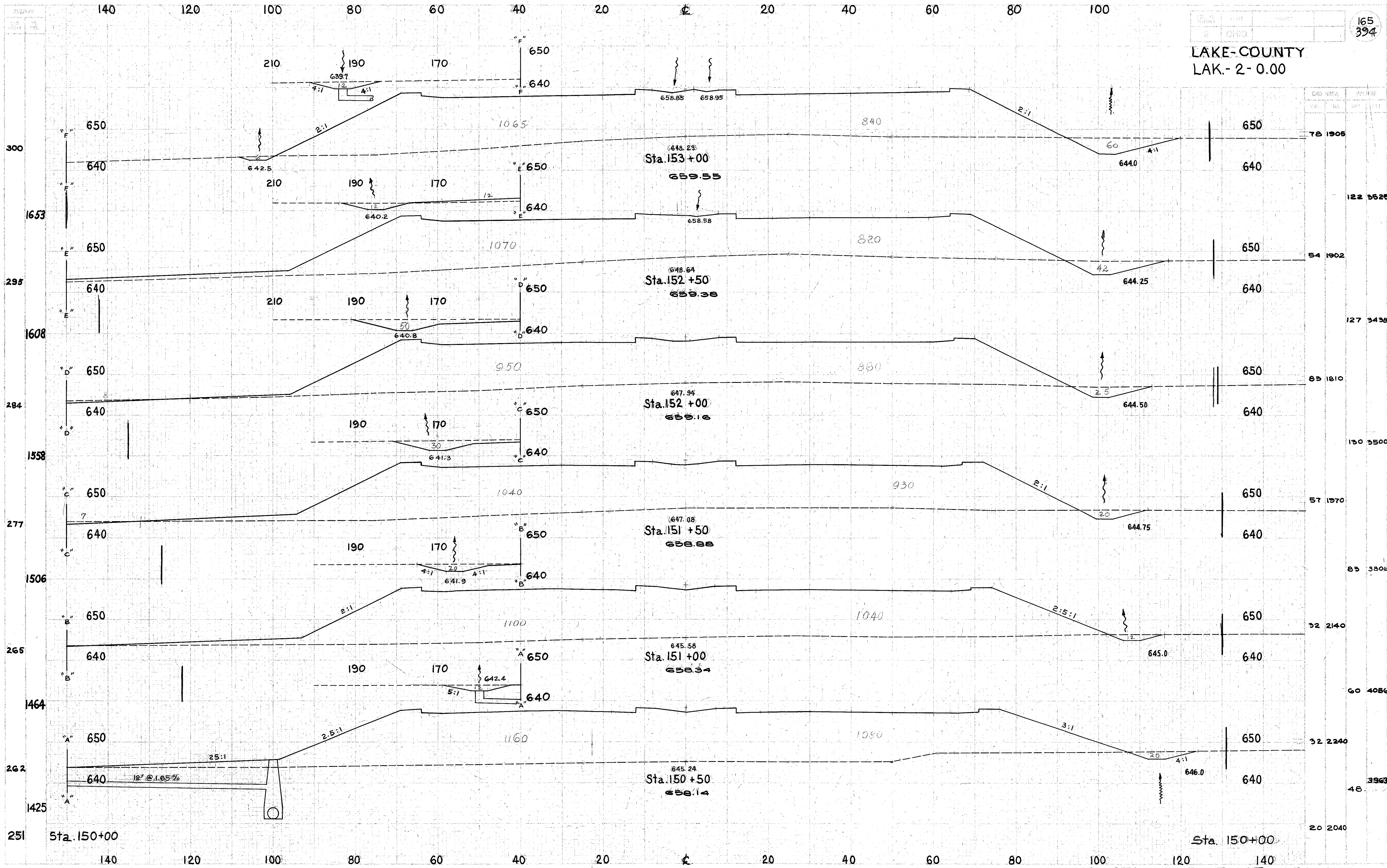
CROSS SECTIONS STA. 150+50 TO STA. 153+00
