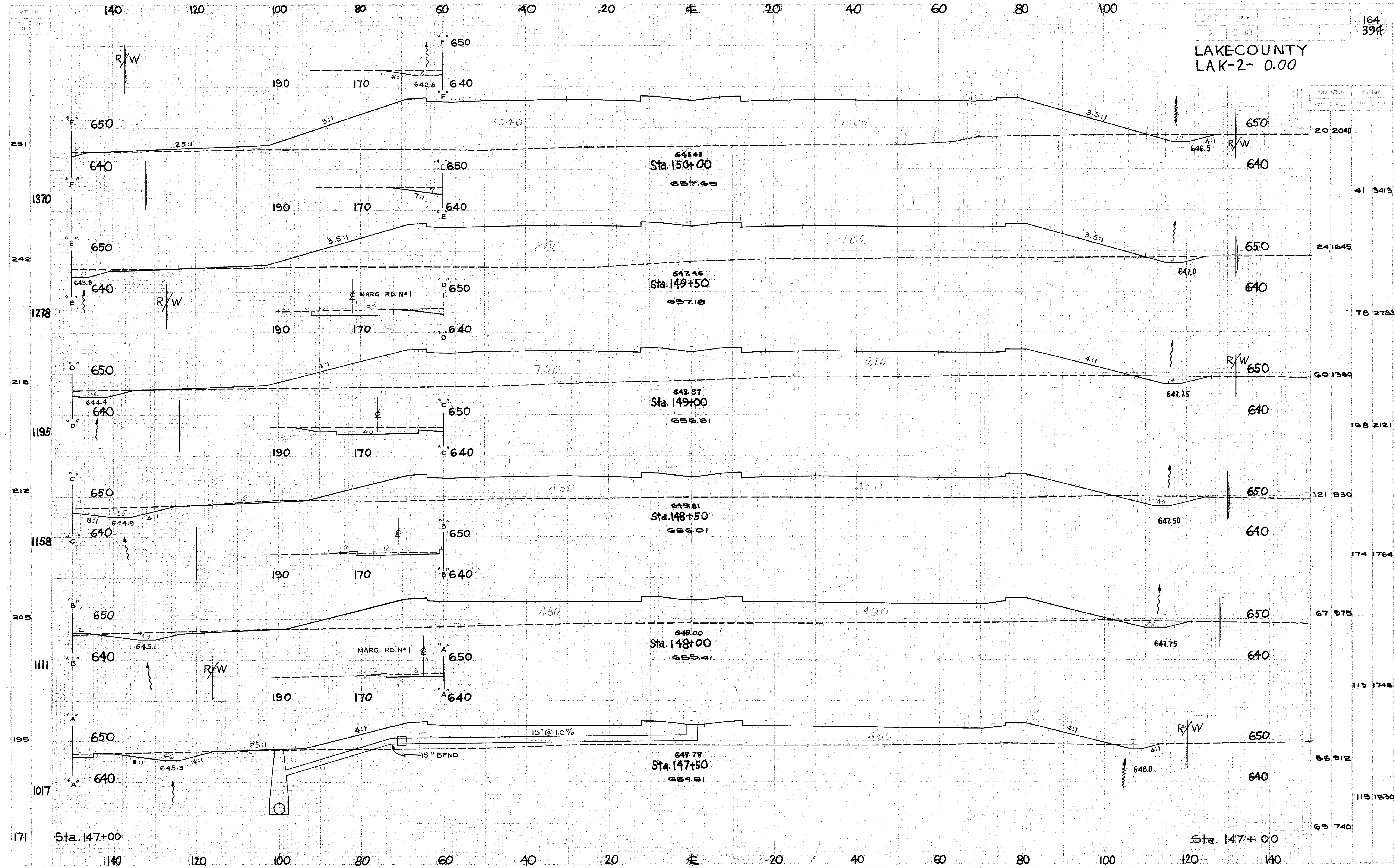
CROSS SECTIONS- STA. 147+50 TO STA. 150+00
