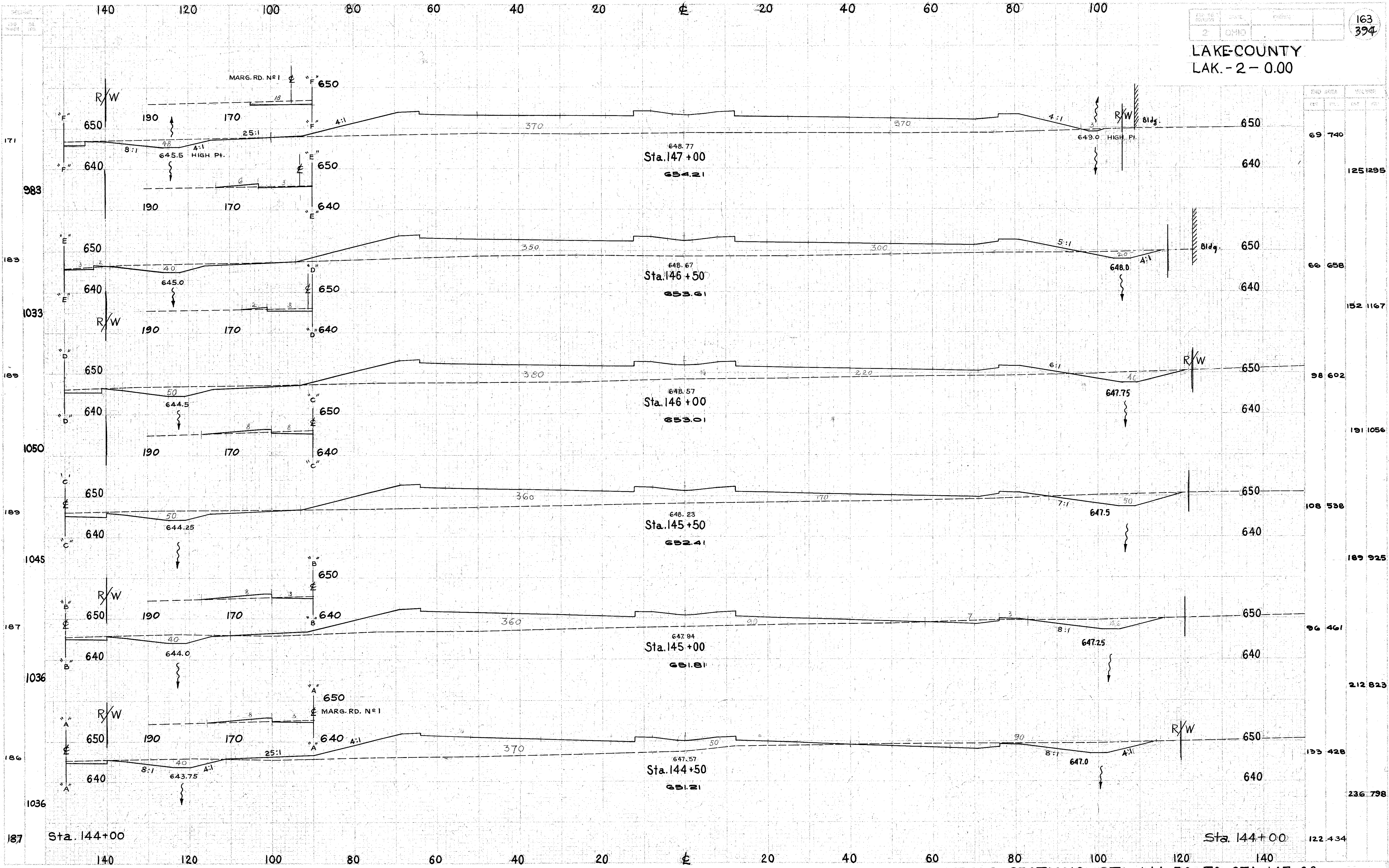
CROSS SECTIONS STA. 144+50 TO STA. 147+00
