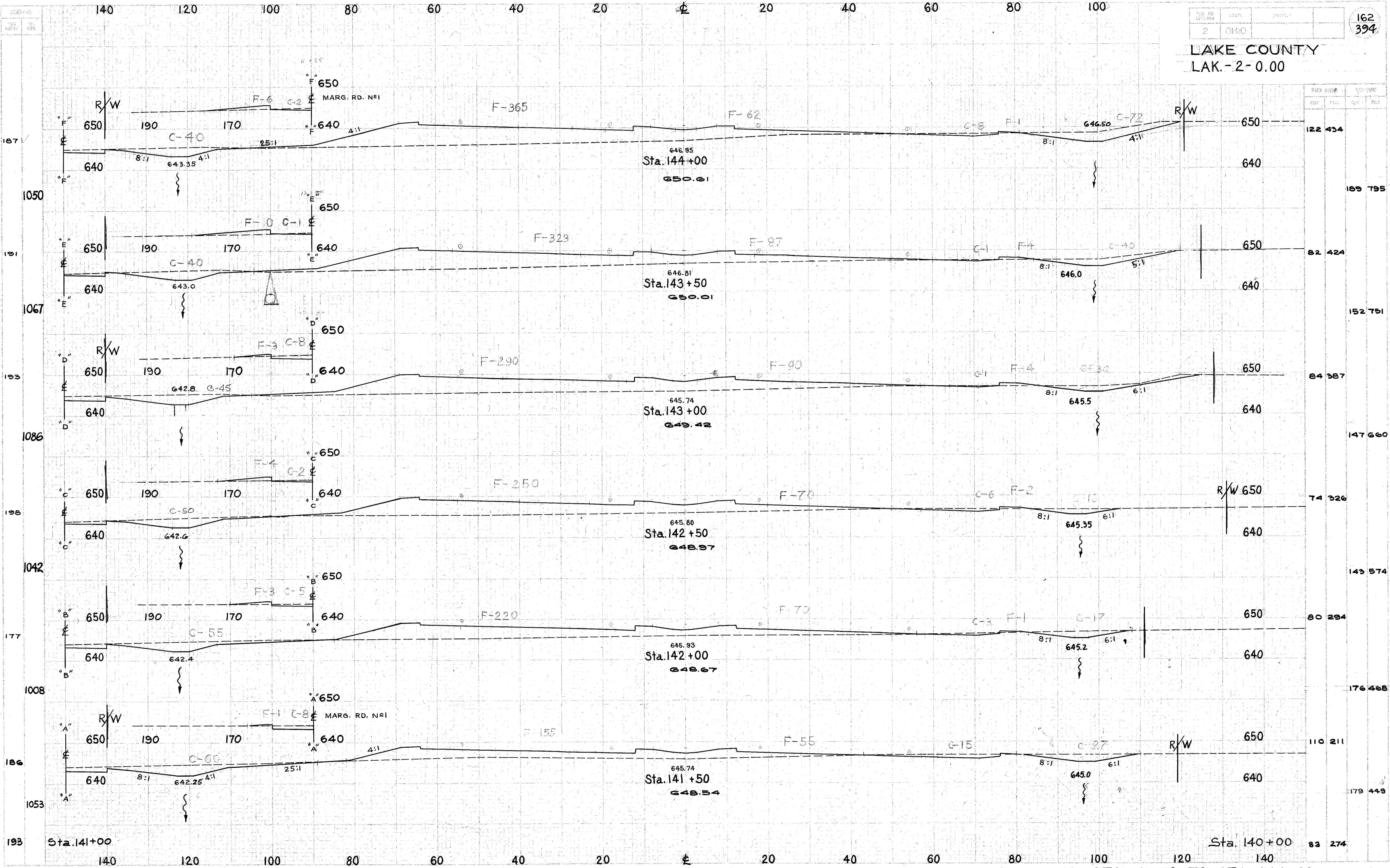
CROSS SECTIONS STA. 141+50 TO STA. 144+00
