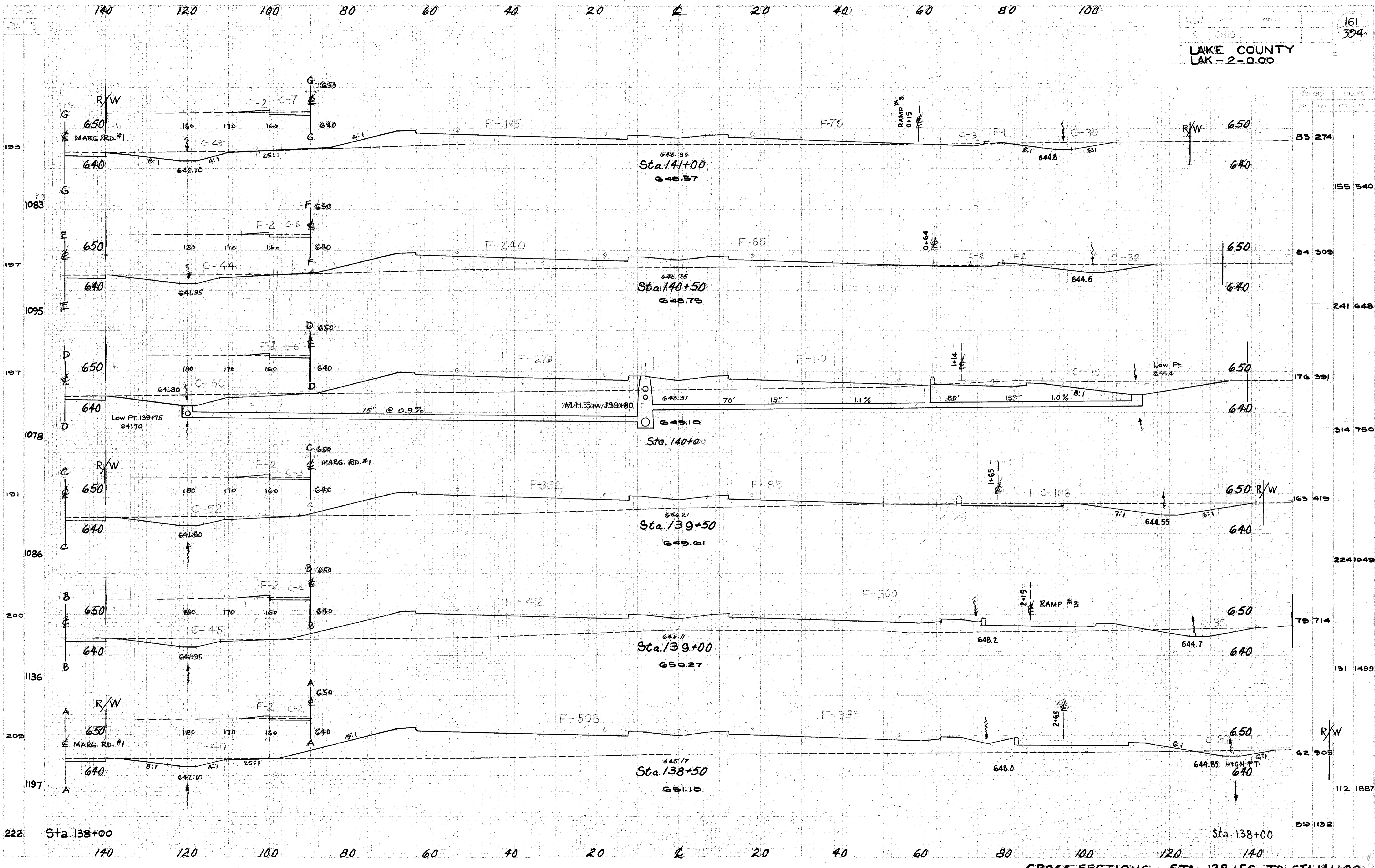
CROSS SECTIONS - STA. 138+50 TO STA. 141+00
