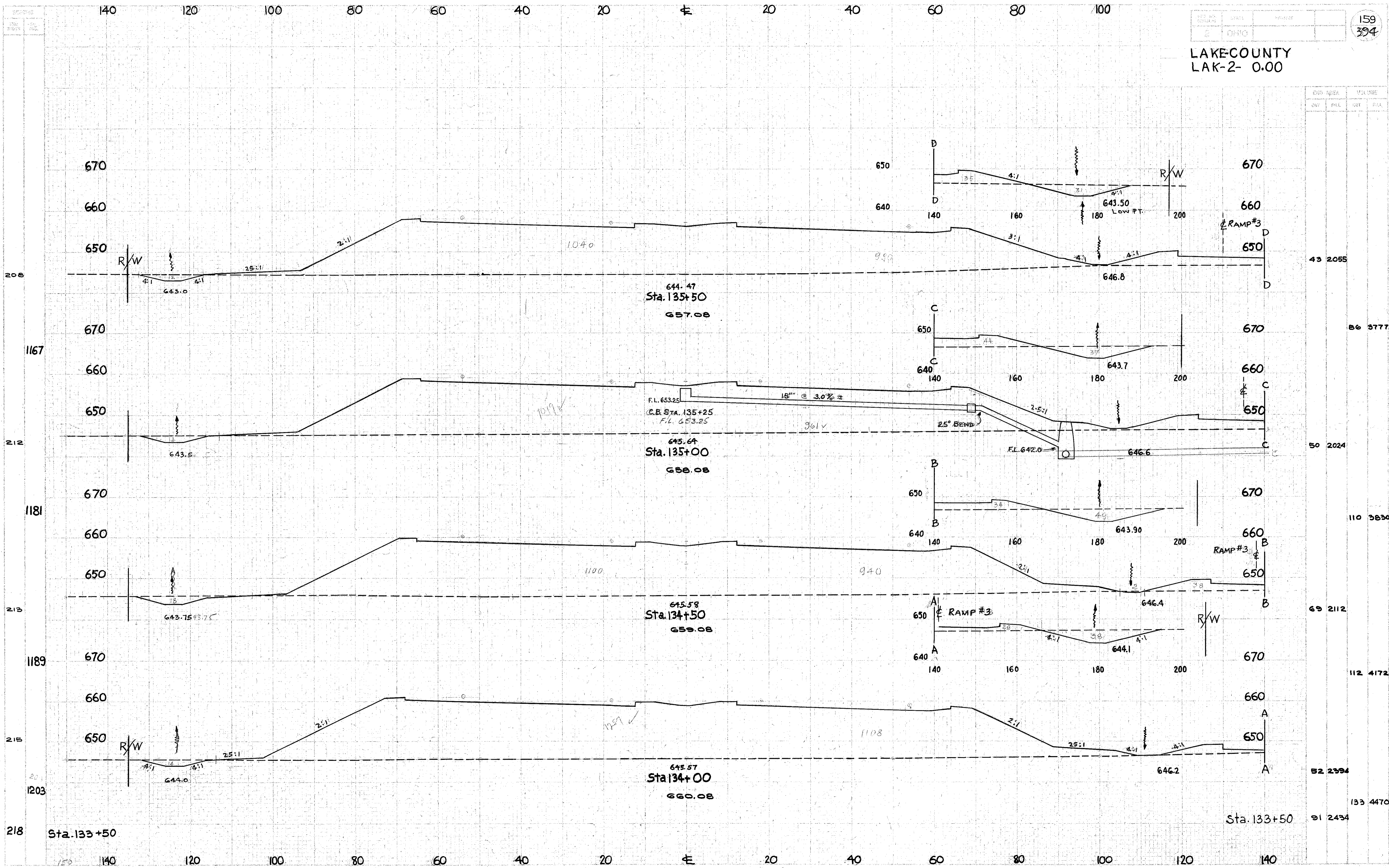
CROSS SECTIONS- STA. 134+00 TO STA. 135+50
